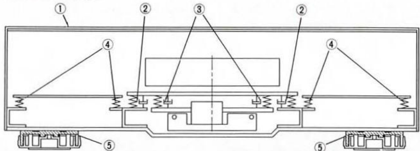
① Contenitore a doppio strato ② Isolatore della meccanica: gomma ③ Isolatore ibrido: gomma e molle a spirale ④ Isolatore della piastra circuitale ⑤ Piedino isolatore in resina termoplastica all'elastomero di poliestere
