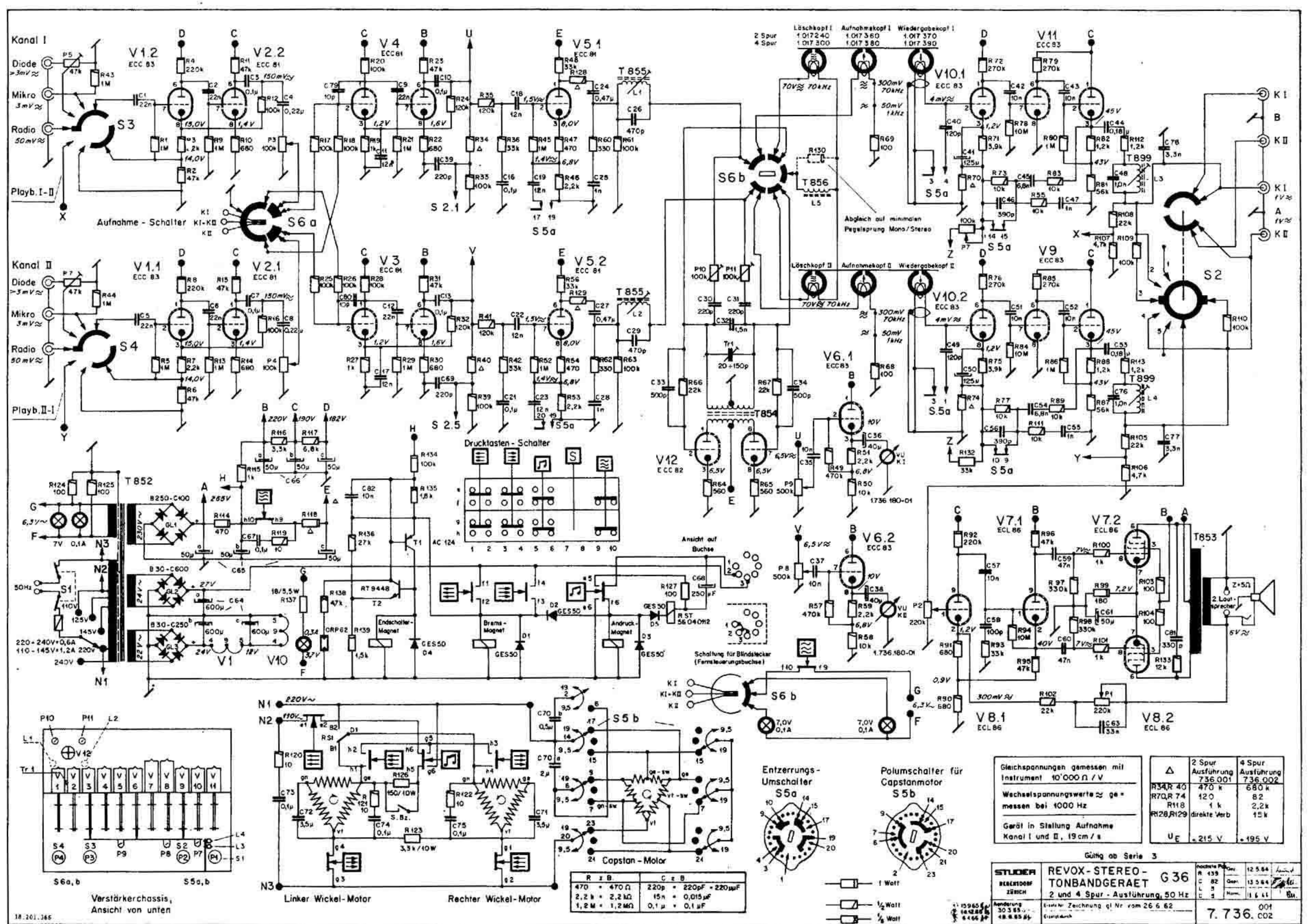
Fig. 7. — Schéma du magnétophone REVOX G 36.
