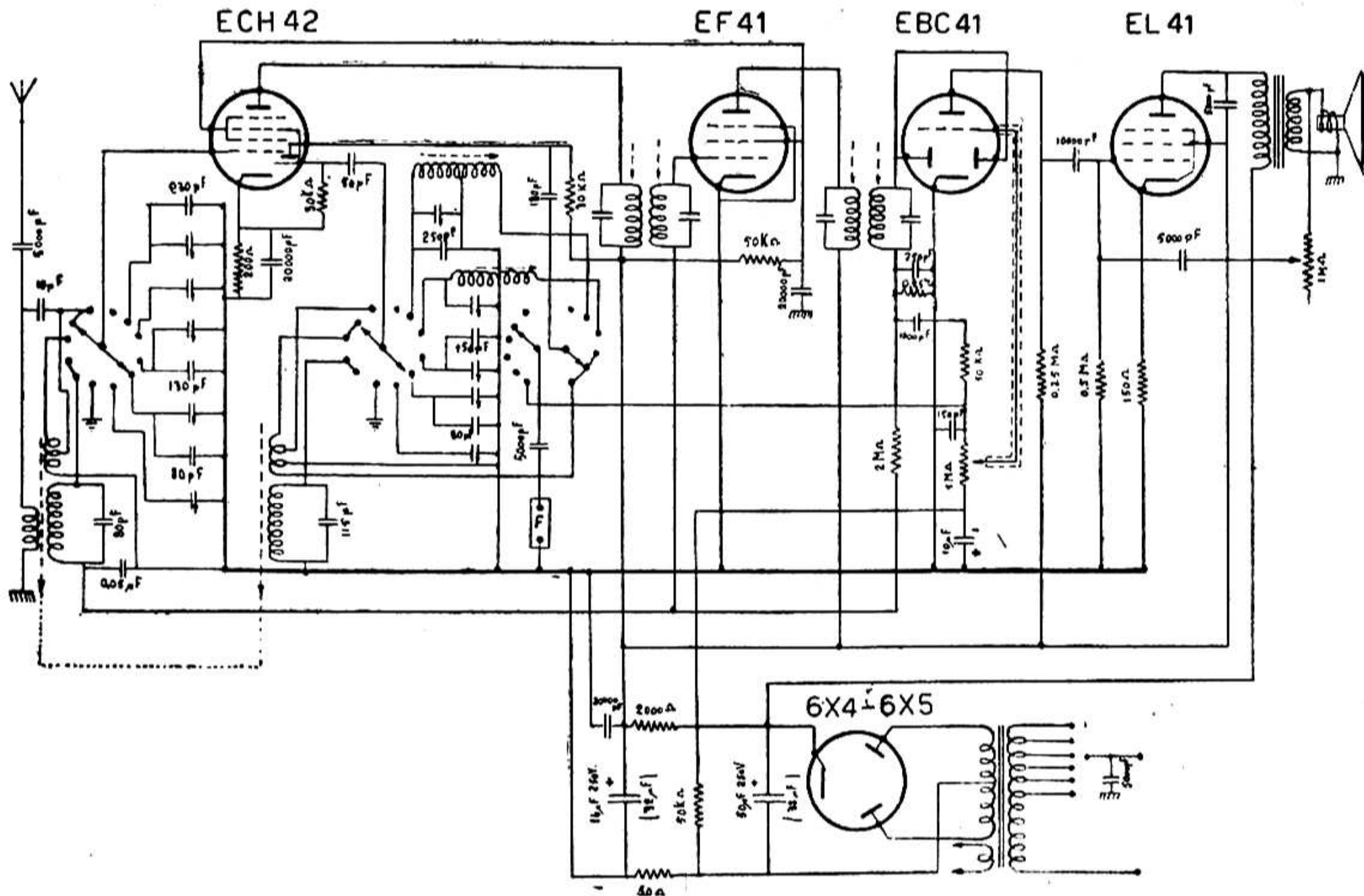
ABC RADIOCOSTRUZIONE - Modd. R 952 e R 953 - Medie e quattro espansioni di gamma in onde corte. Media frequenza 465 kc. Stadio finale con reazione inversa. Potenza d'uscita 3,5 watt.
