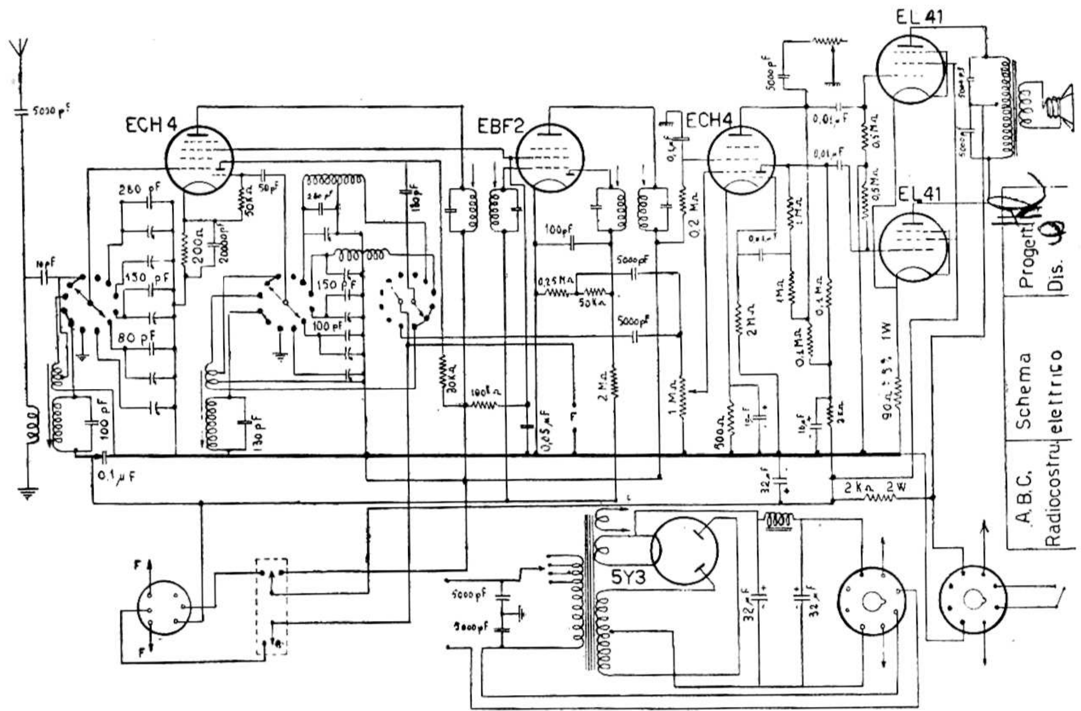
ABC RADIOCOSTRUZIONI - Mod. 972 (il mod. R 972/FM è eguale, con in più il sintonizzatore FM a cinque valvole) - Sintonia a permeabilità variabile e doppia espansione di gamma. La seconda ECH4 provvede alla preamplificazione BF e all'inversione di fase. Potenza d'uscita 4,5 watt indistorti.
