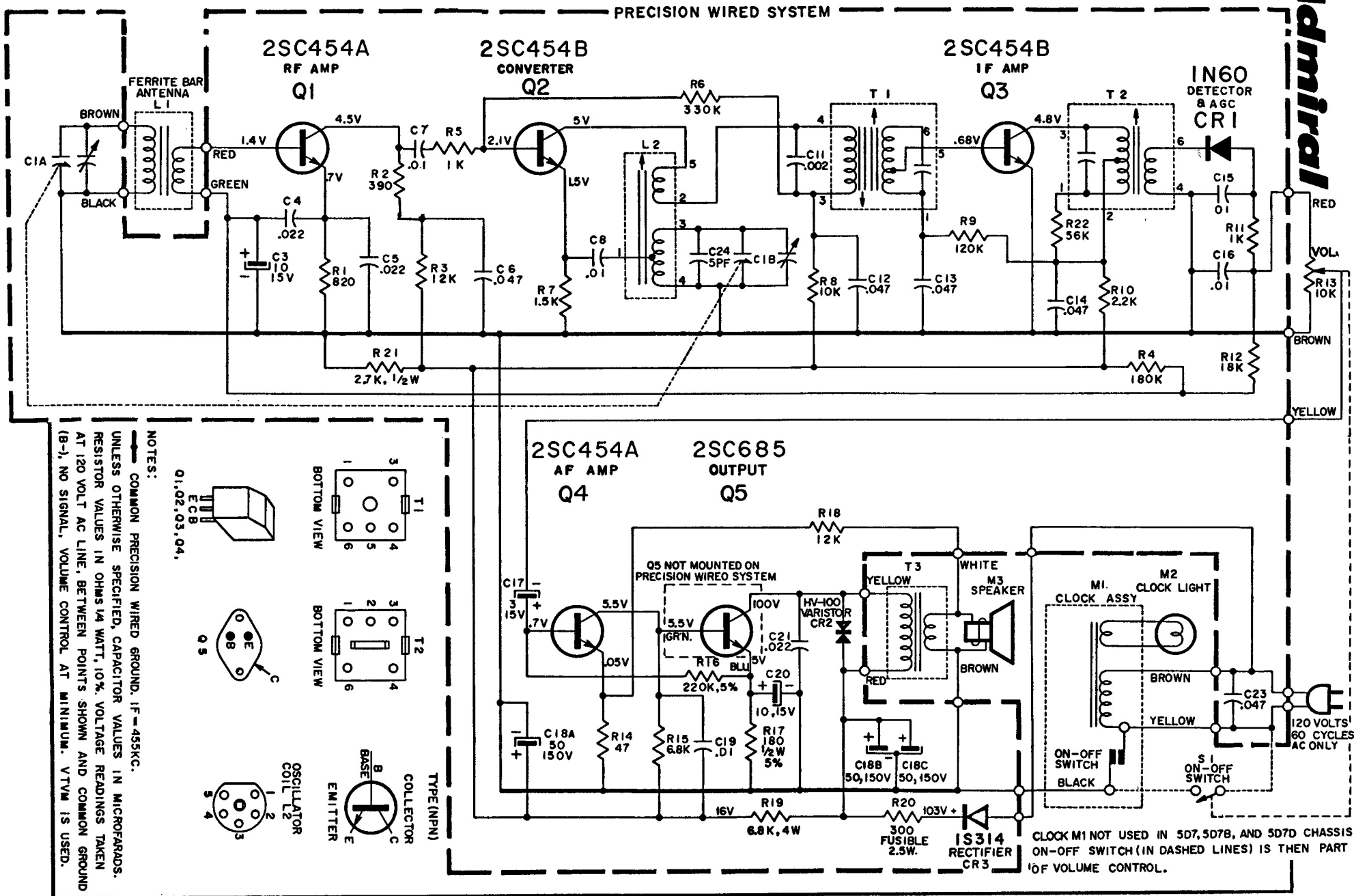
5D7, 5D7A, 5D7B, 5D7C, 5D7D, 5D7E SCHEMATIC DIAGRAM
