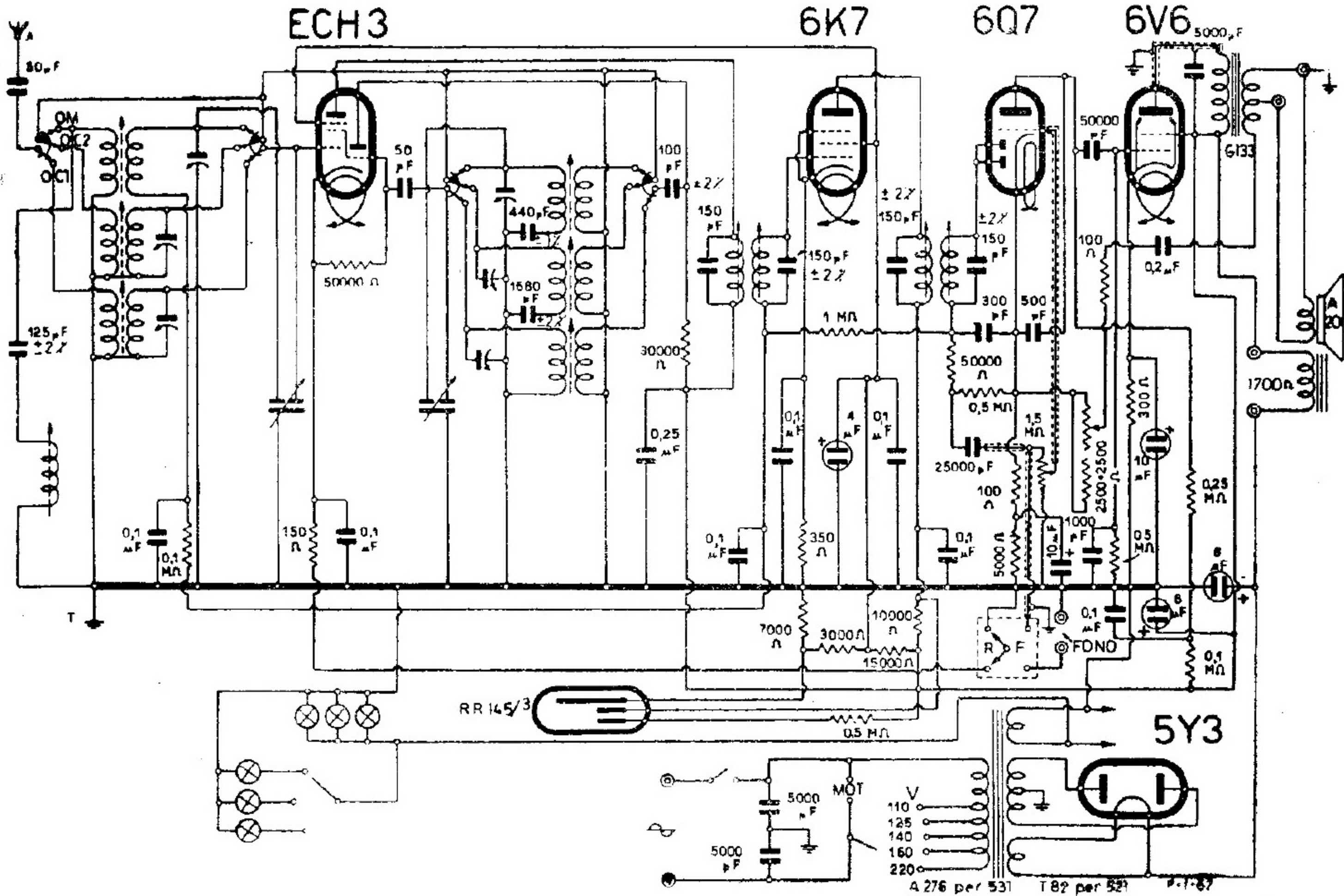
ALLOCCIO, BACCHINI & C. - MODD. « 521 », « 531 », « 534 »
