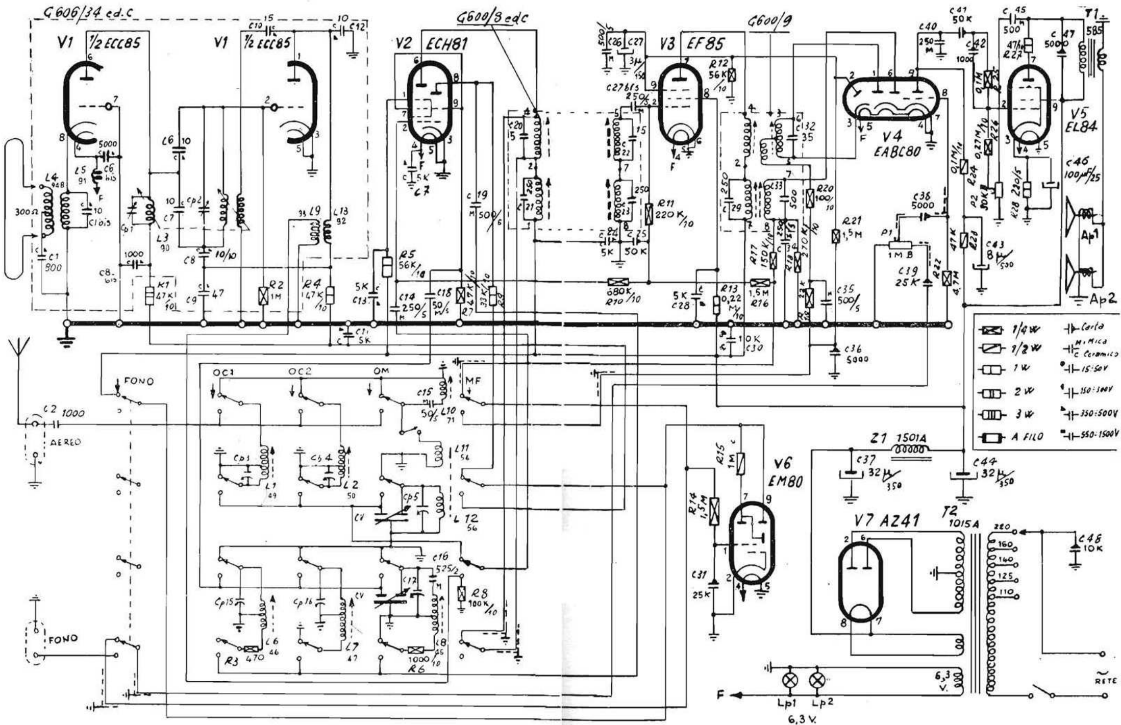
ALLOCCHIO BACCHINI - Mod. 962 MF. Apparecchio a modulazione di ampiezza e di frequenza, con quattro gamme di ricezione, una OM, due OC e una UC a FM. Media frequenza AM a 465 kc/s, e FM a 10,7 Mc/s. Potenza d'uscita 4,5 watt, pot. assorbita 60 VA.
