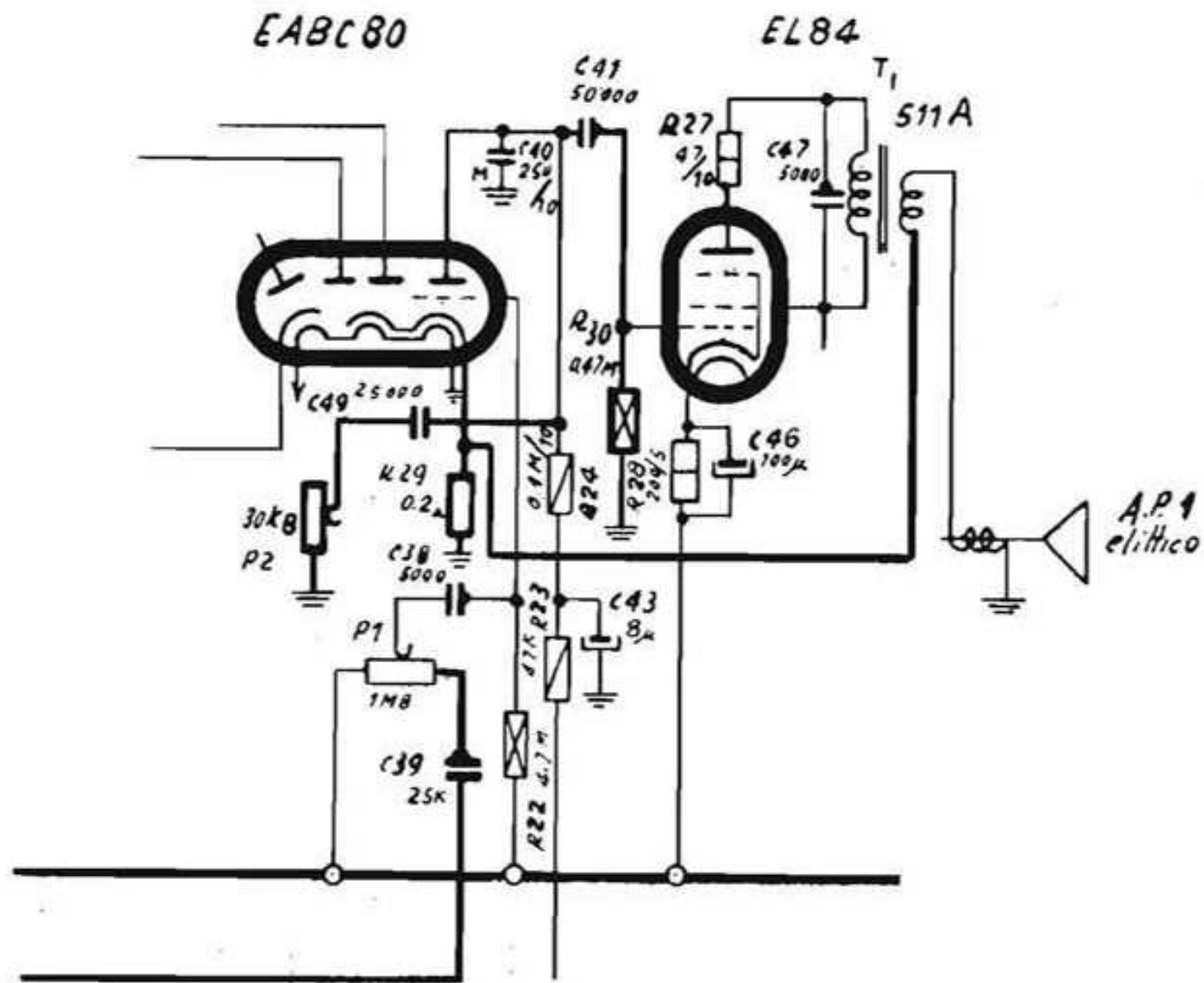
ALLOCCHIO BACCHINI - Mod. 961 - Variante dello stadio finale, il resto dello schema è quello dell'apparecchio mod. 962 MF.
