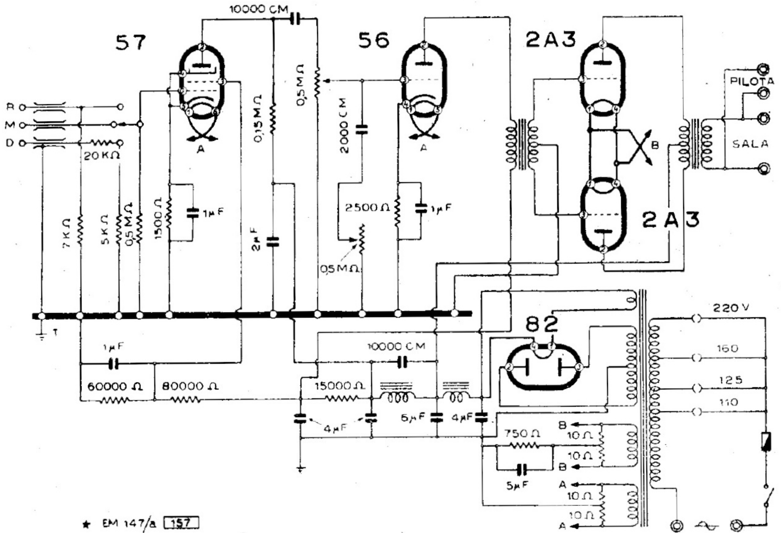
ALLOCCIO, BACCHINI & C. - AMPLIFICATORE MOD. «ALBI 12 - I Serie»
