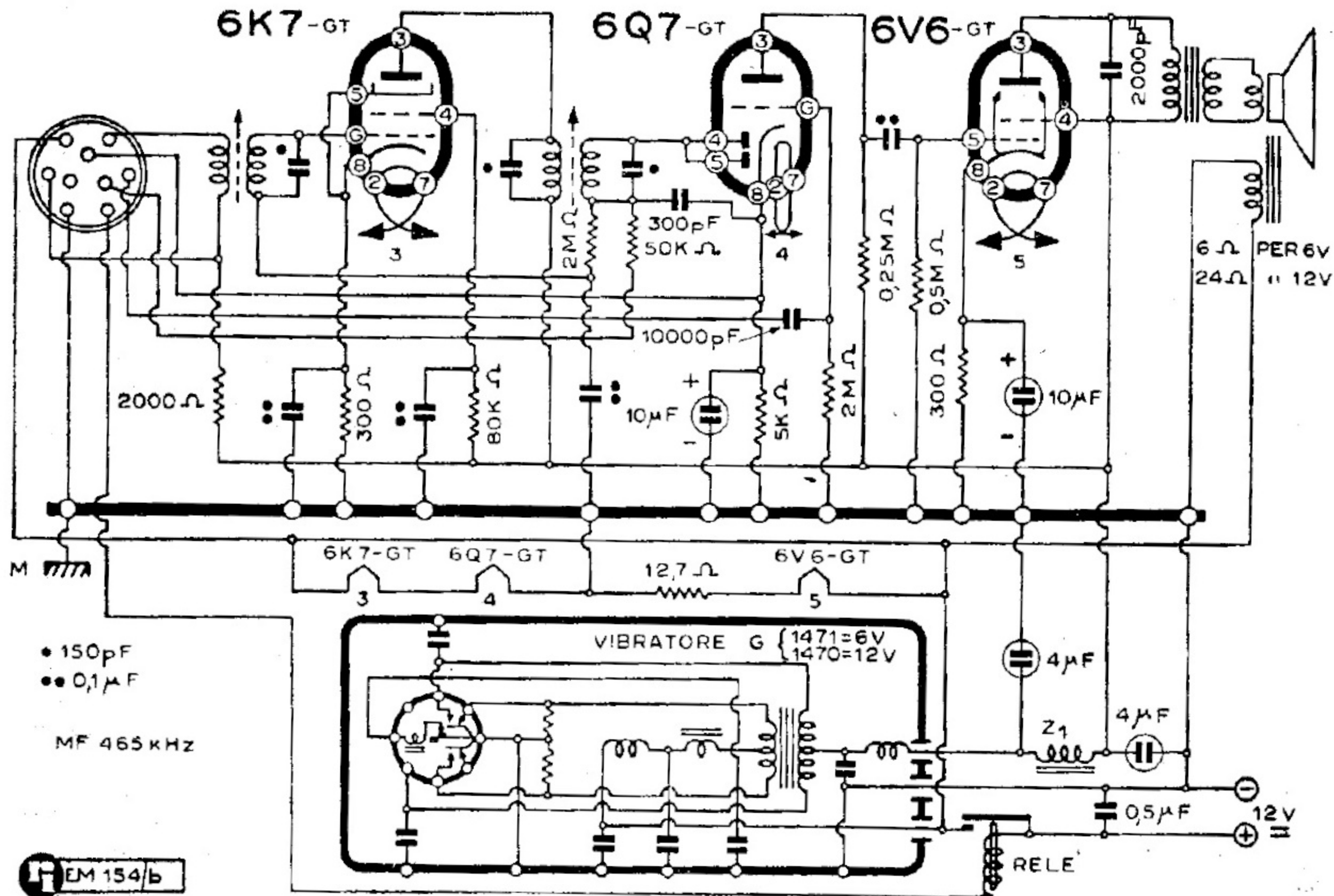
ALLOCCHIO, BACCHINI & C. - MOD. « AUTONOLA IV/3W », BF, MF, ALIM.
