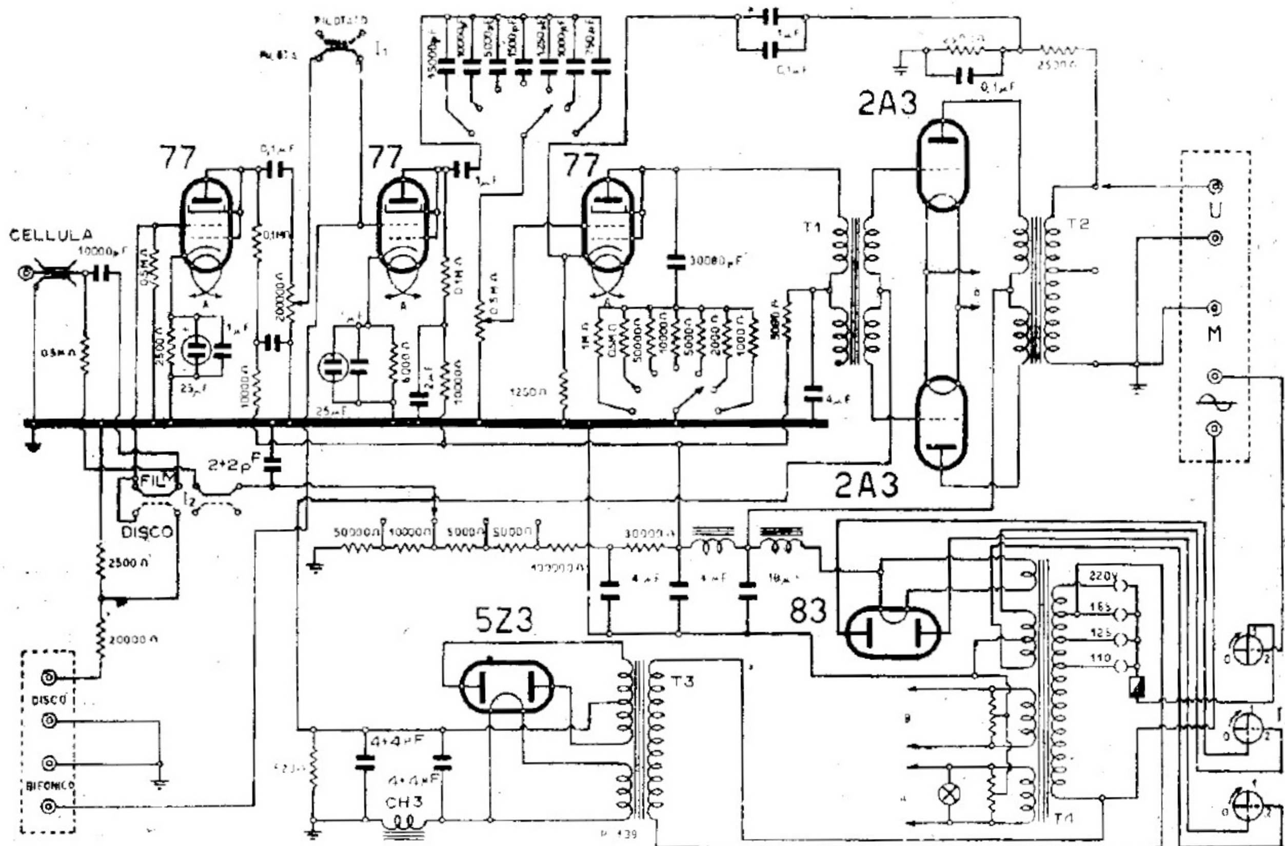
ALLOCCIO, BACCHINI & C. - AMPLIFICATORE MOD. « D 45 P »
