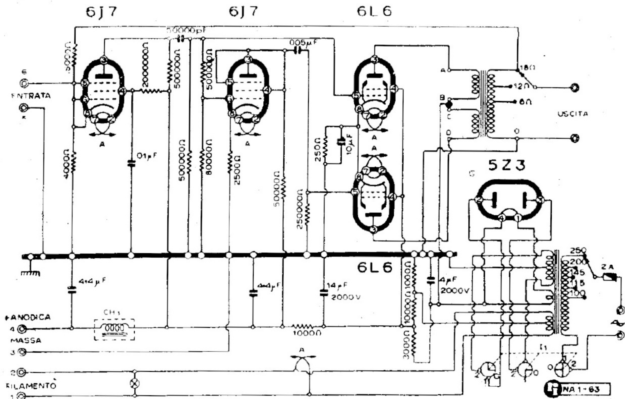
ALLOCCHIO, BACCHINI & C. - AMPLIFICATORE MOD. « D 55 »
