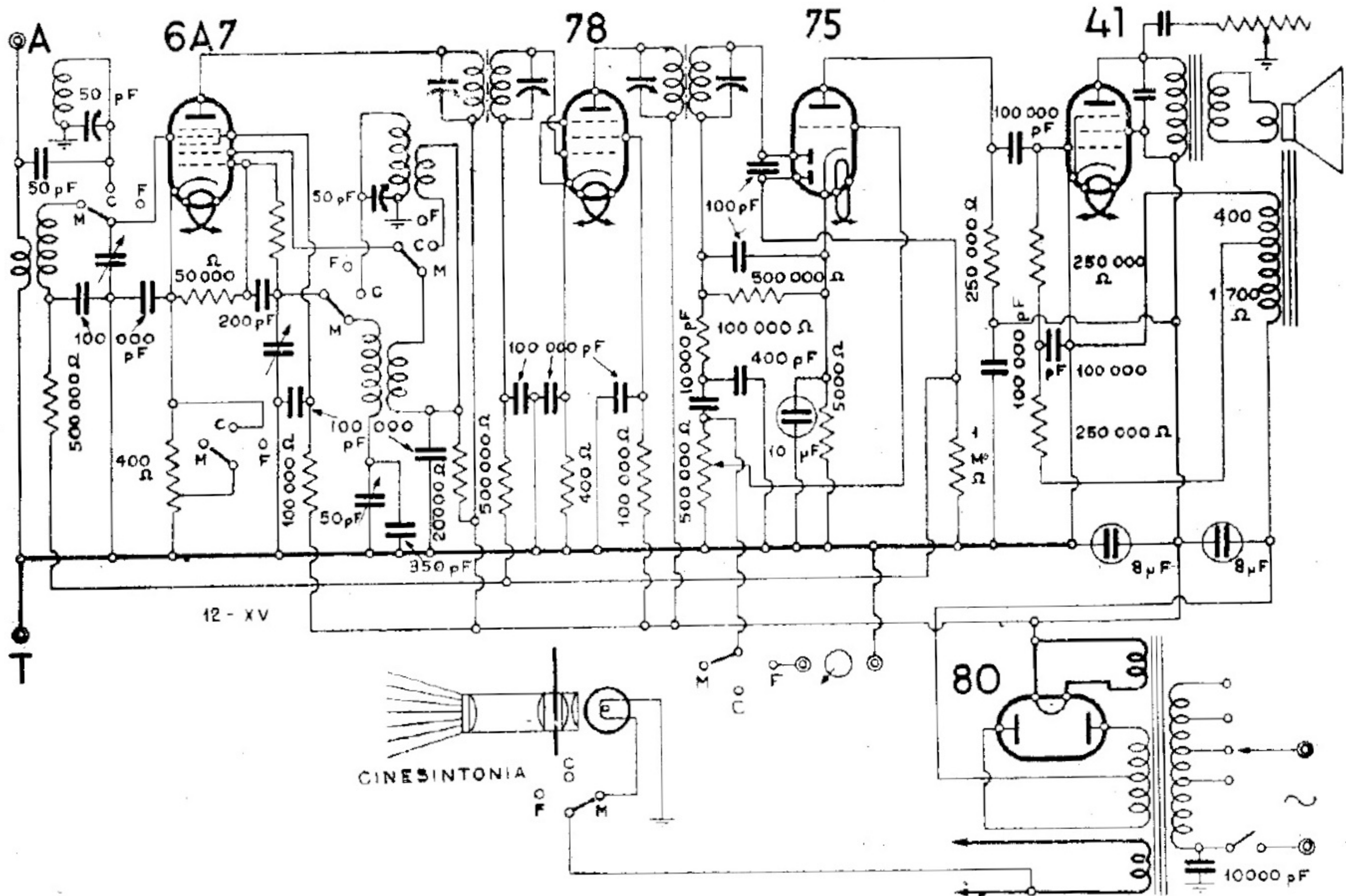
AREL - MODD. « 5 VALVOLE » - « ECO DEL MONDO » - « ECOFONO »
