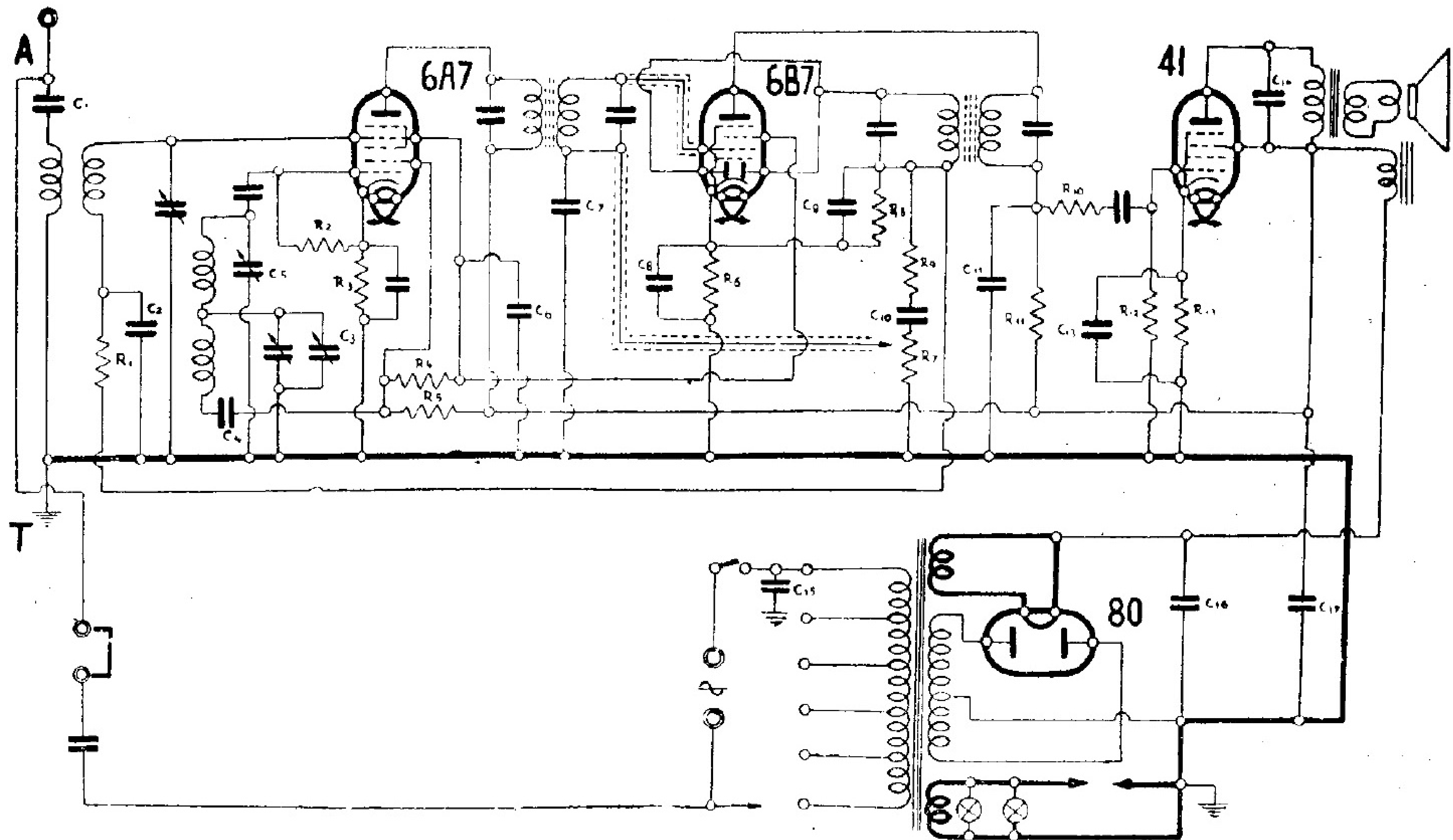
AREL - MOD. « LUMERADIO 1939 »
