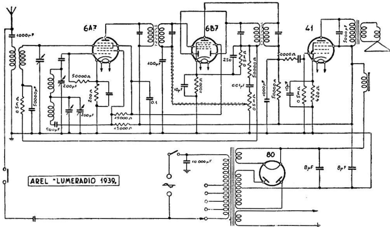
AREL. — Mod. « Lumeradio ». — Produzione 1938-39. — Media frequenza: 450 kHz.
