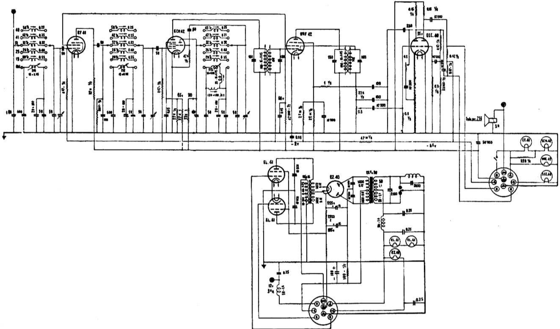
ASTER RADIO - Modd. 746 e 756 - Apparecchi radio da automobile, adatti per pullman. Due finali in controfase. Onde medie e quattro bande. Lunghezze d'onda 19, 25, 31, 41 e 49 metri. Potenza d'uscita media 10 watt.
