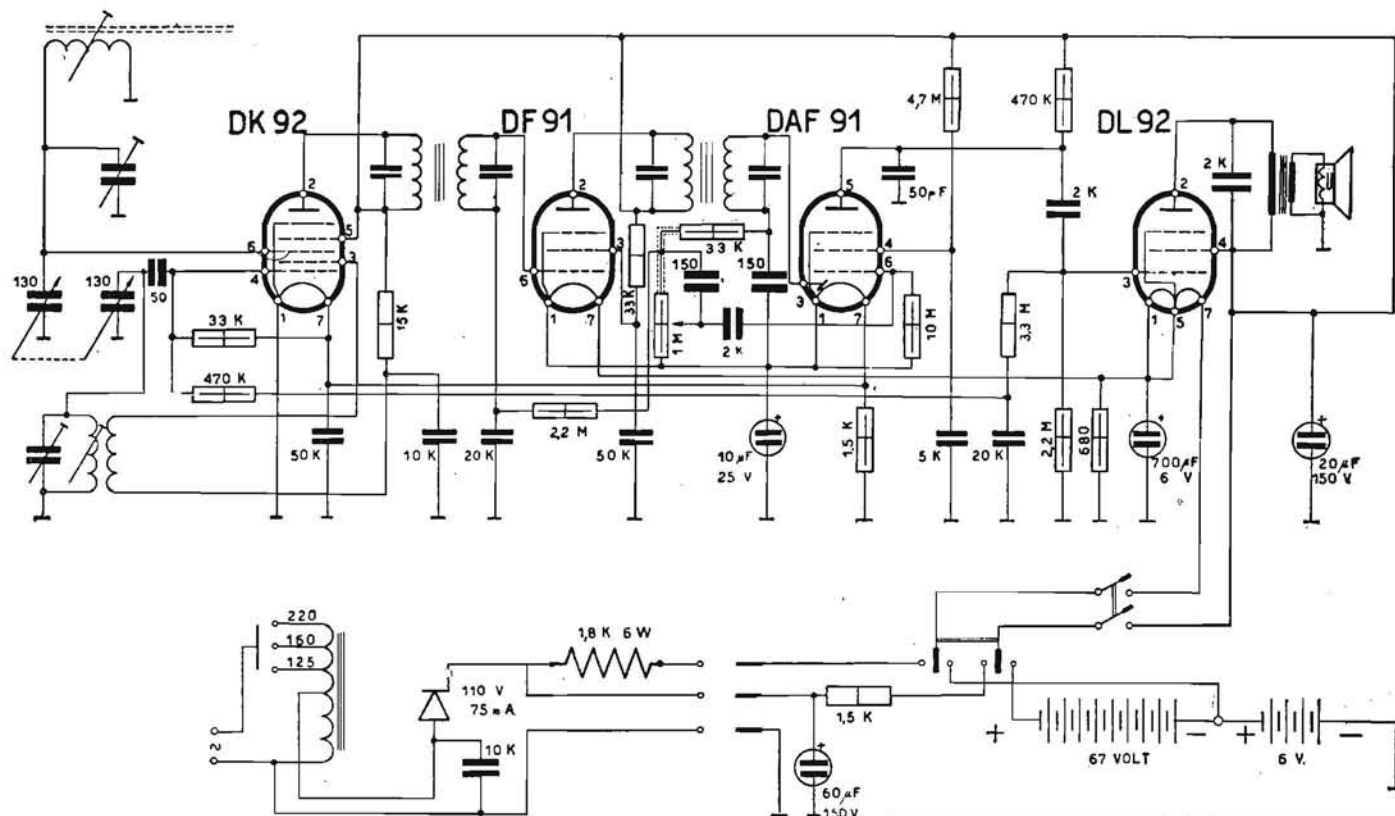
SCHEMA ELETTRICO DEL RADIORICEVITORE PORTATILE AUTOVOX Mod. 411
