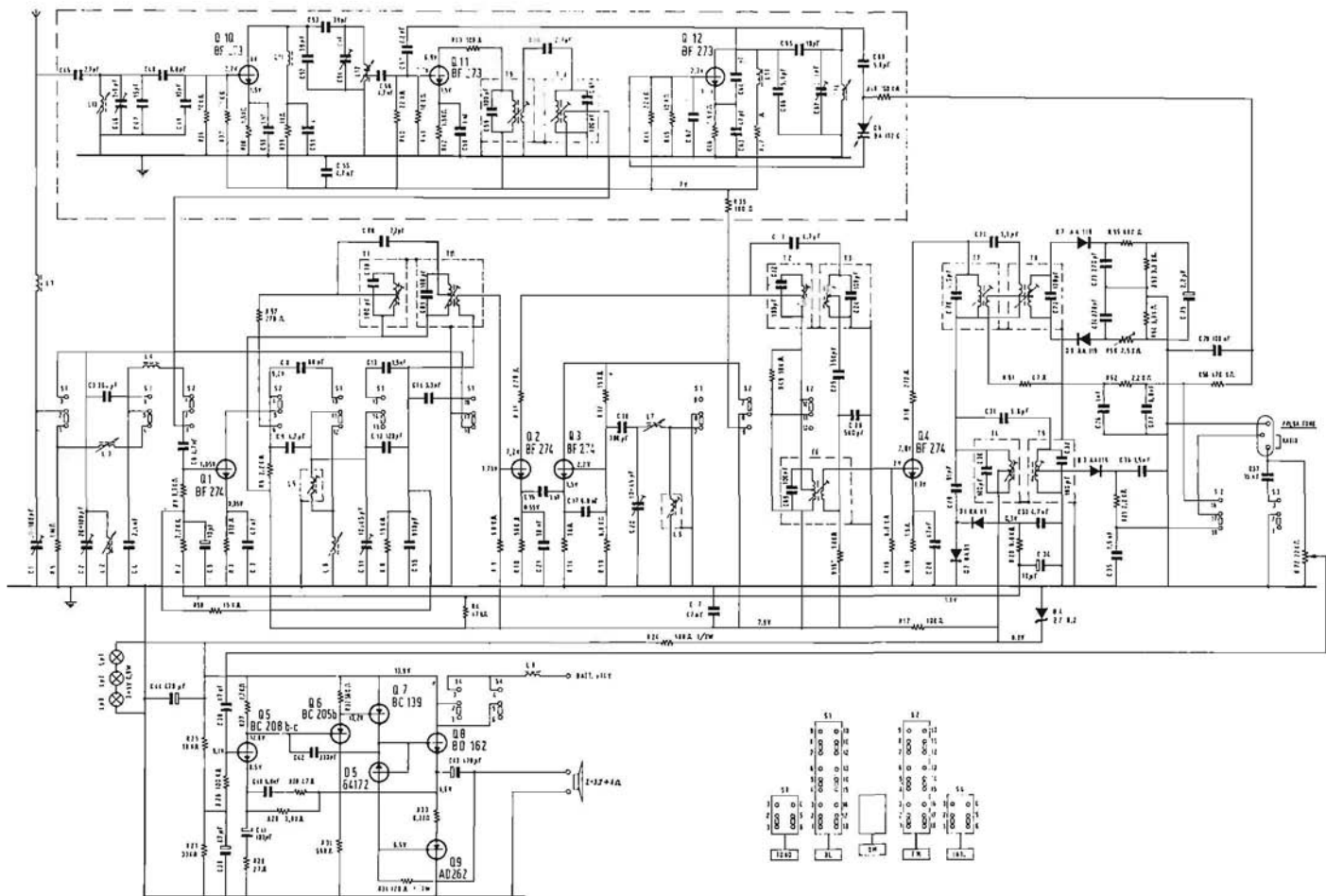
Fig. 3.26. - Schema elettrico di autoradio a tre gamme d'onda: OM-OL-FM. - (Autovox RA/RB277A).
