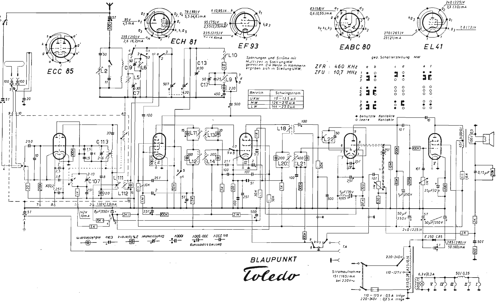
BLAUPUNKT (Blaupunkt Werke GmbH, Hildesheim) - Mod. Toledo. Apparecchio a modulazione d'ampiezza e di frequenza, a tre gamme d'onda, medie e lunghe con antenna in ferrite e ultracorte (FM). MF/AM a 460 kc/s, MF/FM a 10,7 Mc/s. Potenza d'uscita 3 watt. Consumo 45 watt.
