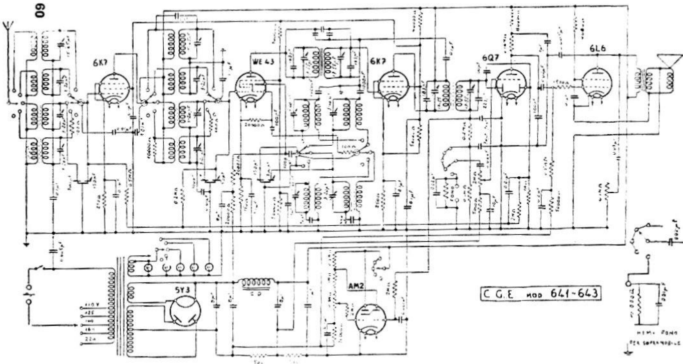
COMPAGNIA GENERALE DI ELETTRICITA. — Mod. 641 e 643 radiofonografo. — Produzione 1933-39. — Media frequenza: 459 kHz.
