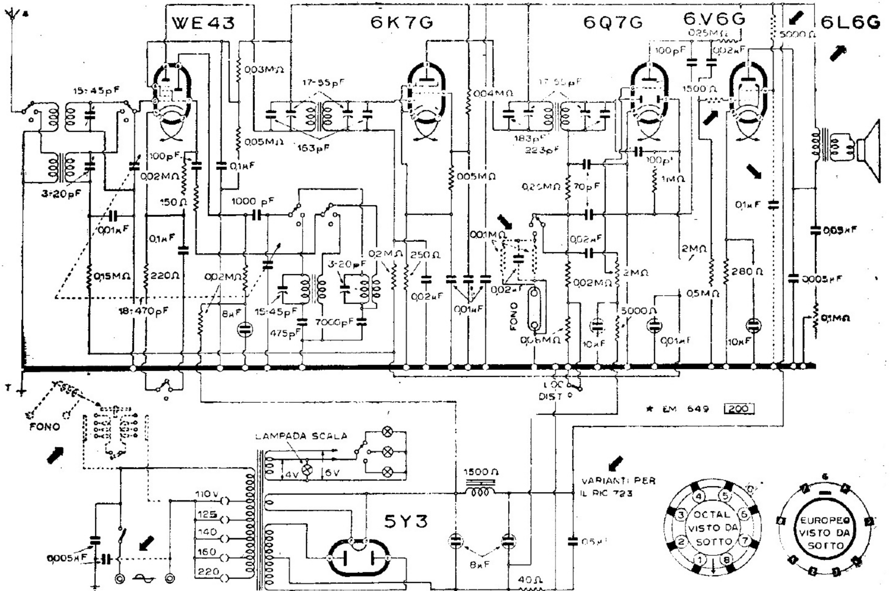
COMPAGNIA GENERALE DI ELETTRICITA' - MOBD. «721» «723»
