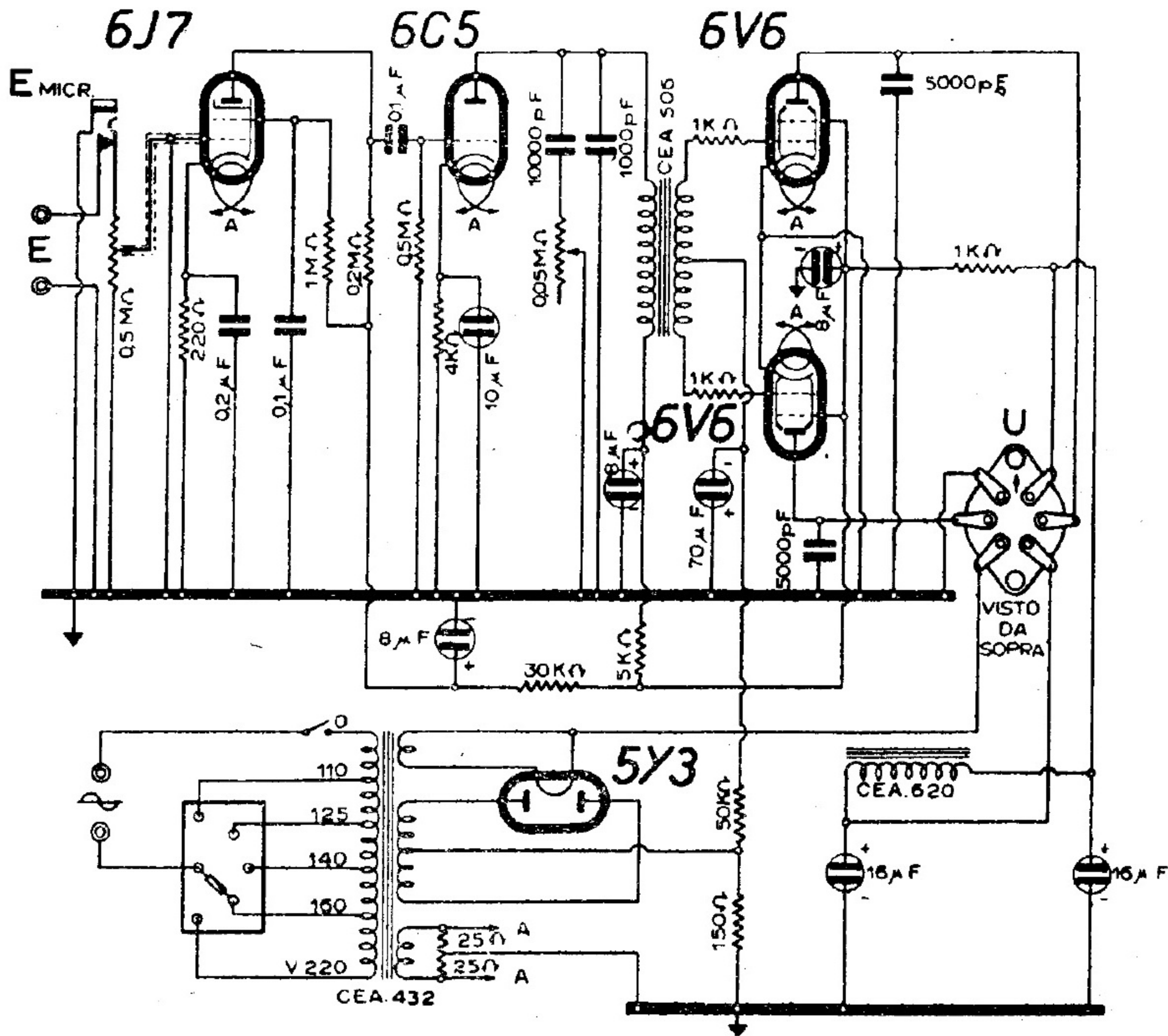
COMPAGNIA GENERALE DI ELETTRICITA' . AMPLIFICATORE MOD. « AP 12 W »
