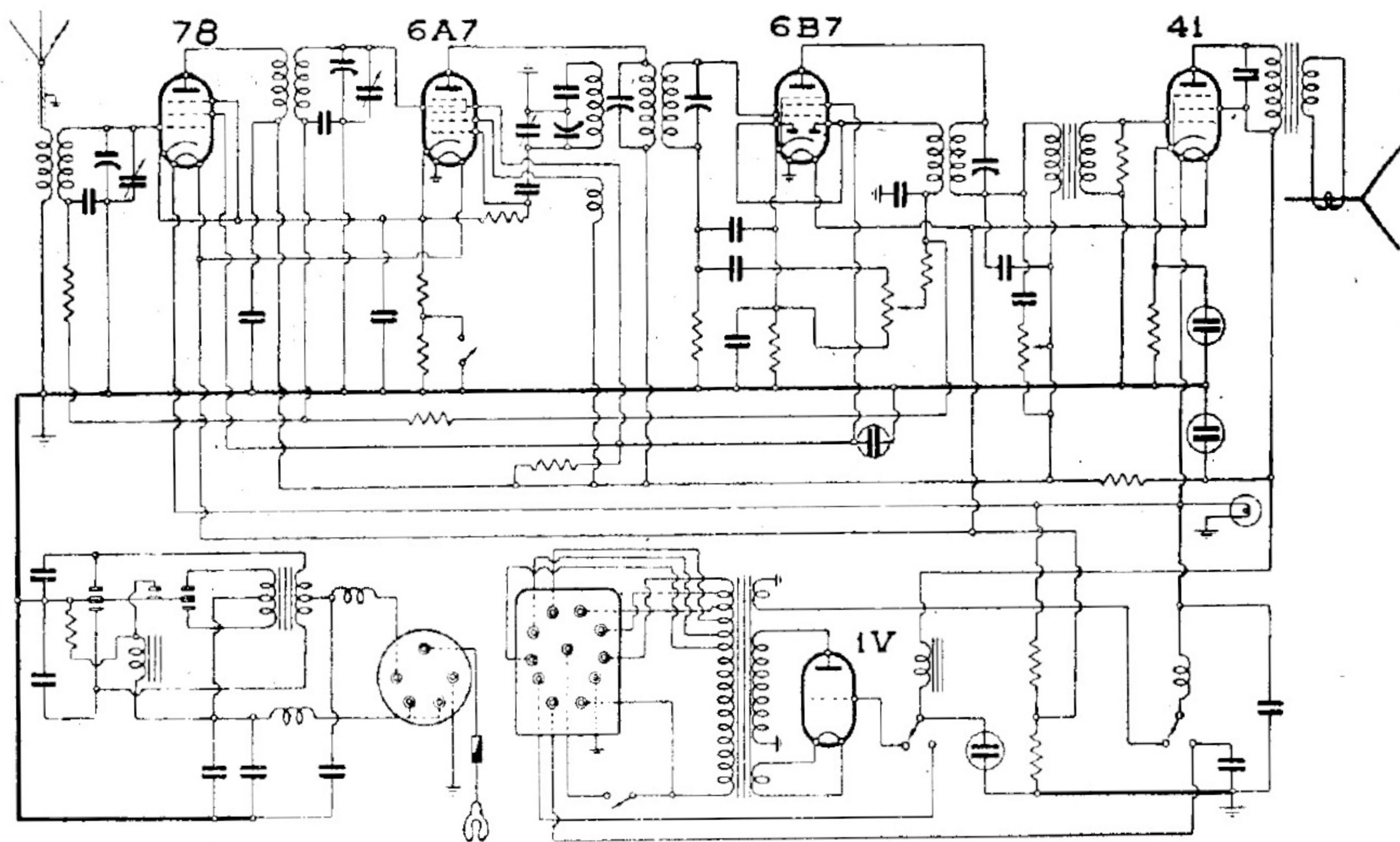
COMPAGNIA GENERALE DI ELETTRICITA' - MOD. « AUTORADIO B. 52 »
