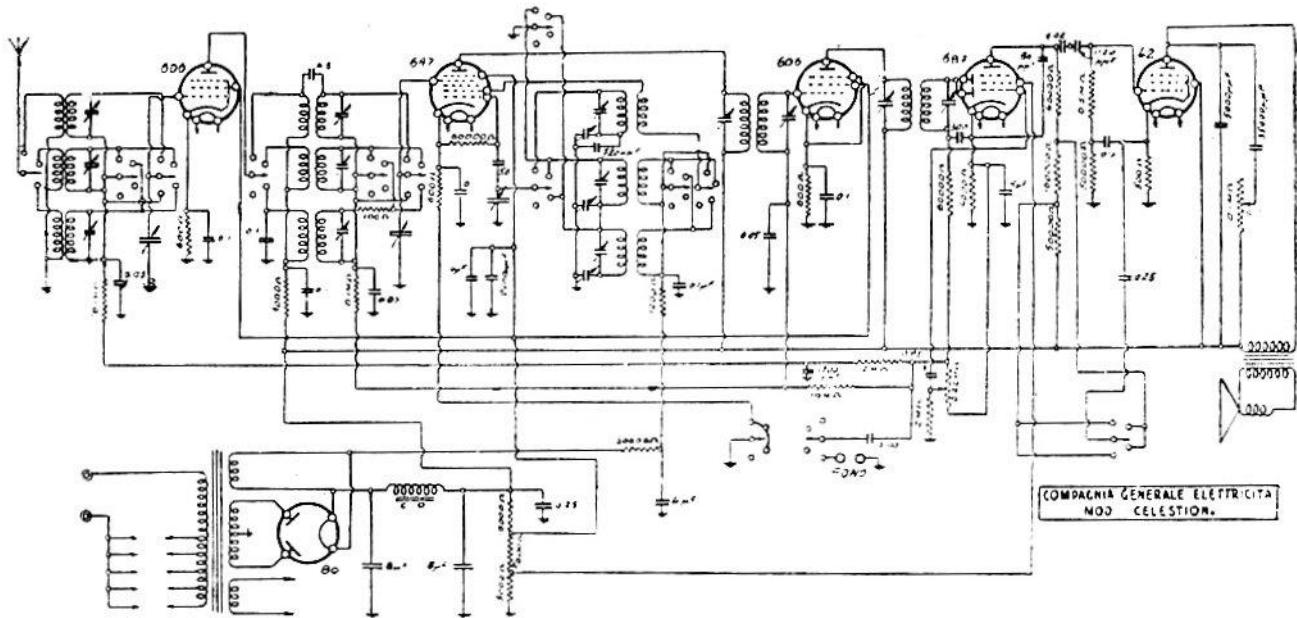
COMPAGNIA GENERALE DI ELETTRICITA. — Modelli: « Celestion trionda, fonotrionda e consol-trionda ». — Produzione 1936. — Media frequenza: 460 kc.
