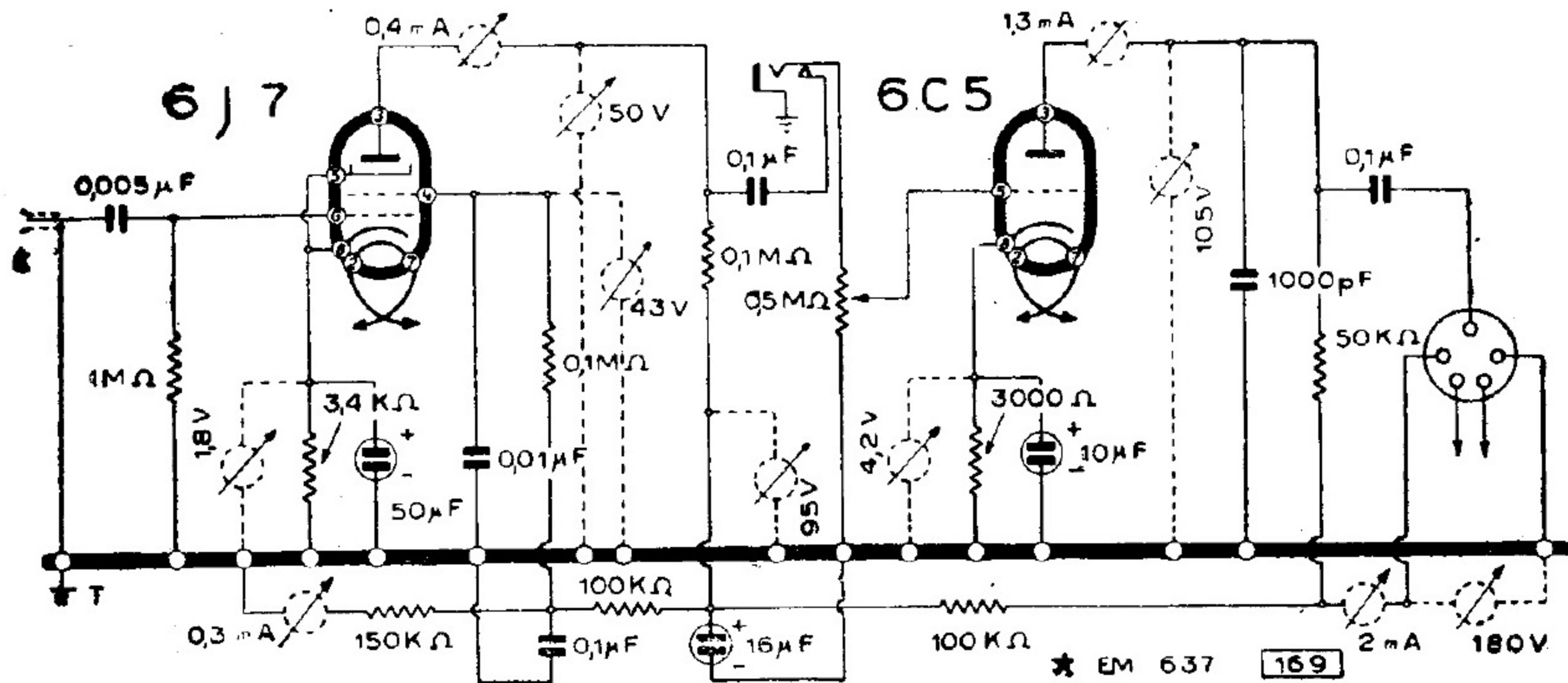
COMPAGNIA GENERALE DI ELETTRICITA' MOD. « PREAMPLIFICATORE A 2 STADI »
