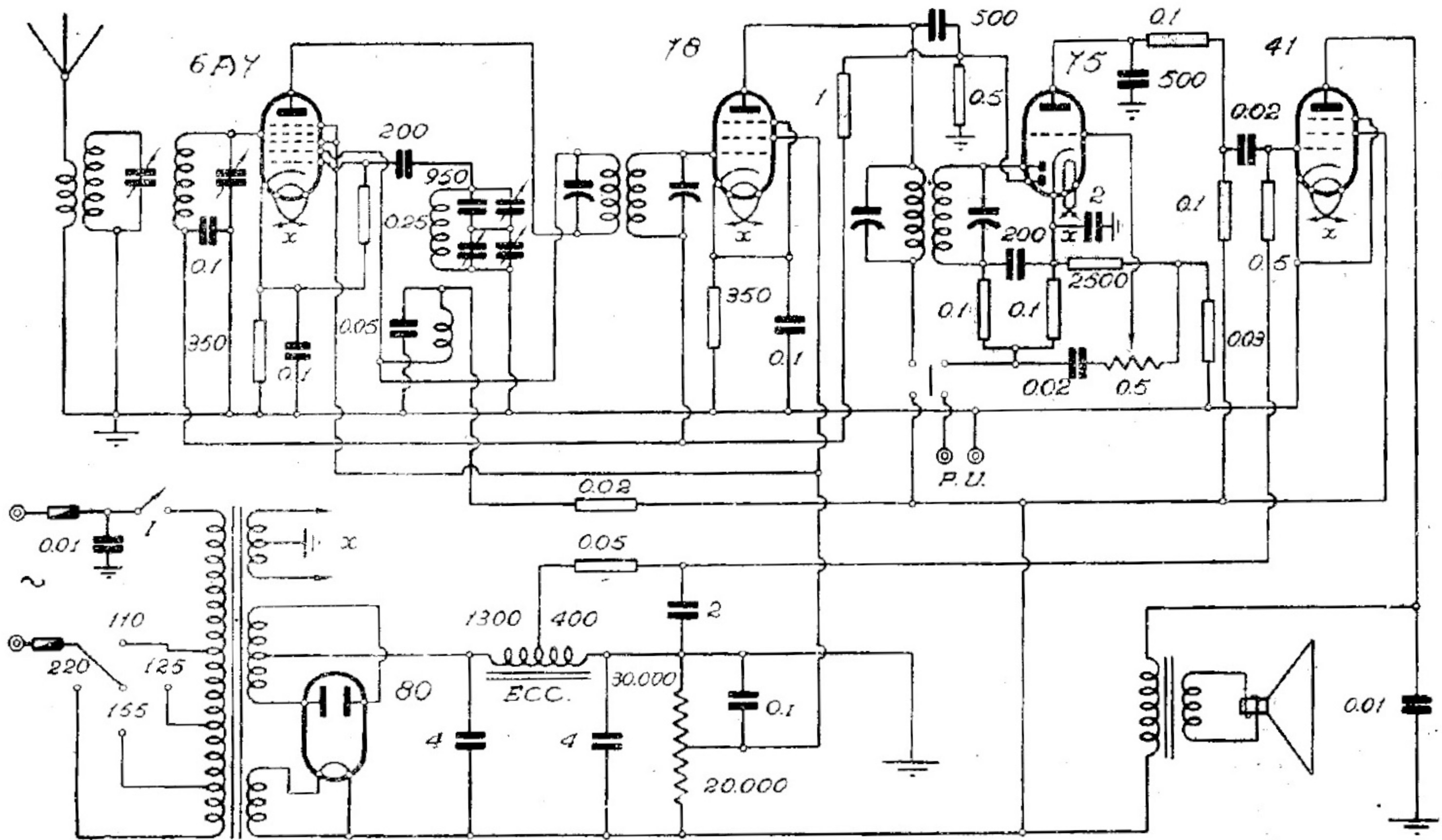
COMPAGNIA GENERALE DI ELETTRICITA' - MOD. « RADIORURALE »
