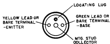
DS 501—Transistor Terminals
