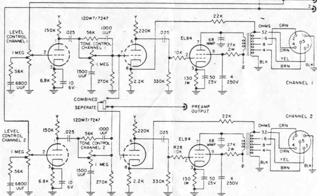
CIRCUITO Nº 55 — Amplificador estereofónico "EICO", mod. AF-4.
