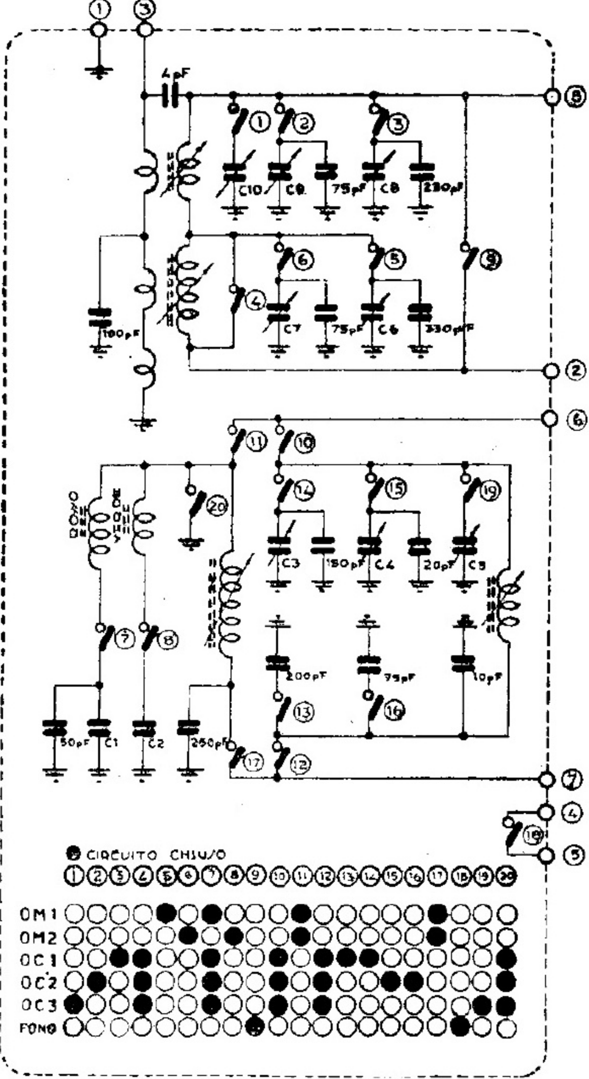
Lo schema elettrico del gruppo P1 Nova.
