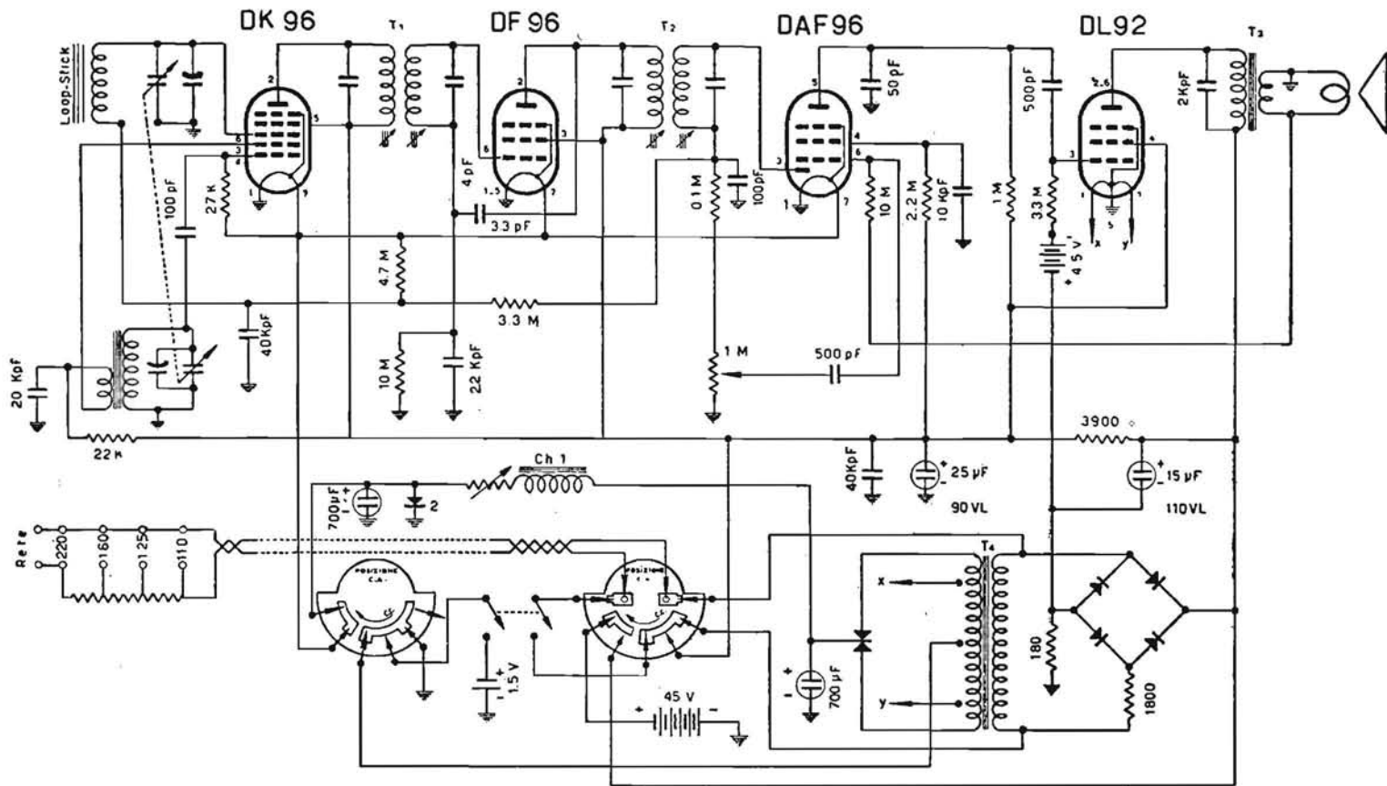
EMERSON-SICART - Mod. Emerson A 737. Apparecchio portatile del tipo pile-rete. L'alimentatore anodico e d'accensione è incorporato. Rettificazione con elementi a selenio. Gamme onde medie con antenna in ferrite. Media frequenza 455 kc/s. Potenza 0,25 watt con pile, 1,2 watt con rete-luce.
