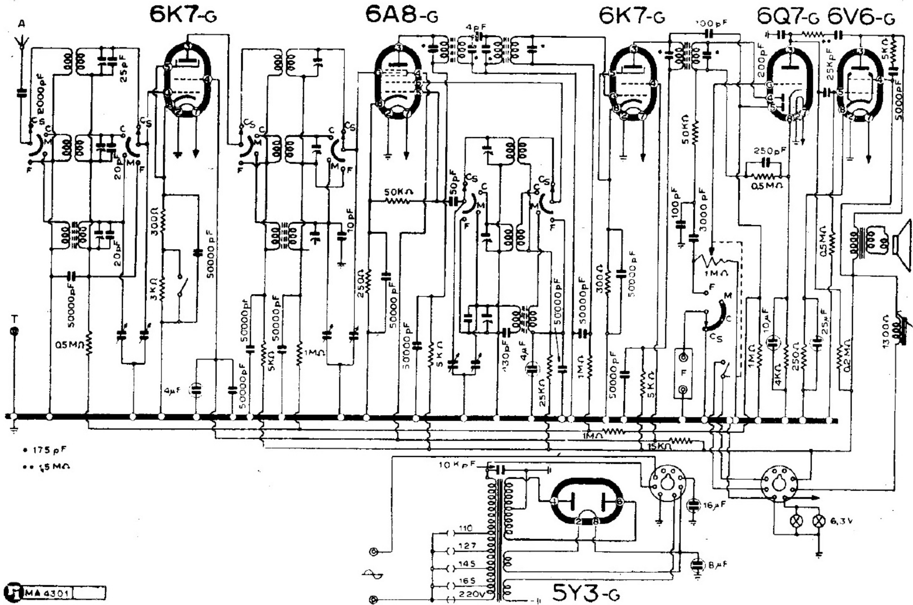
FARA RADIO - MOD. « A 630 »
