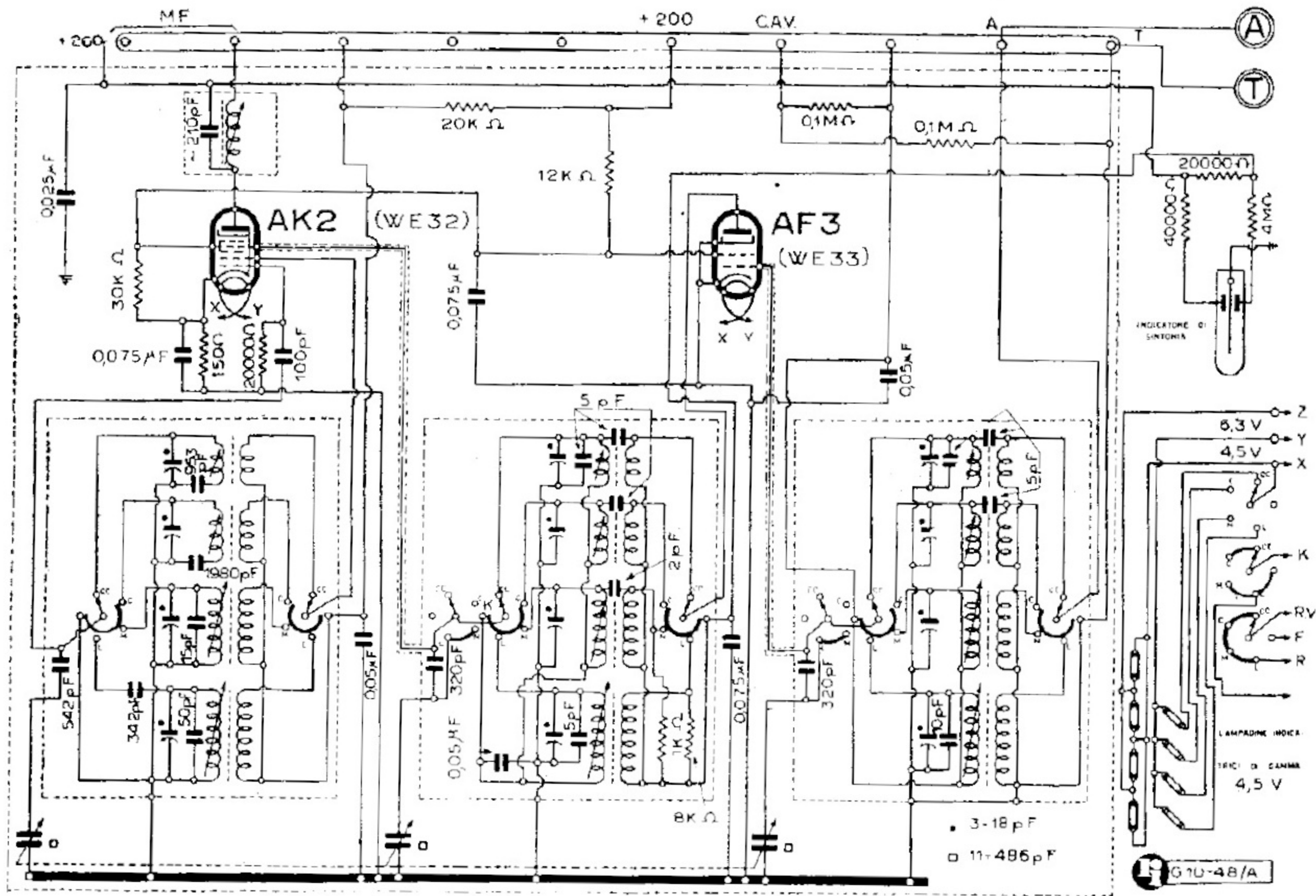
F.I.M.I. - MODD. PHONOLA « 505 » « 506 » - PARTE AF - CONV.
