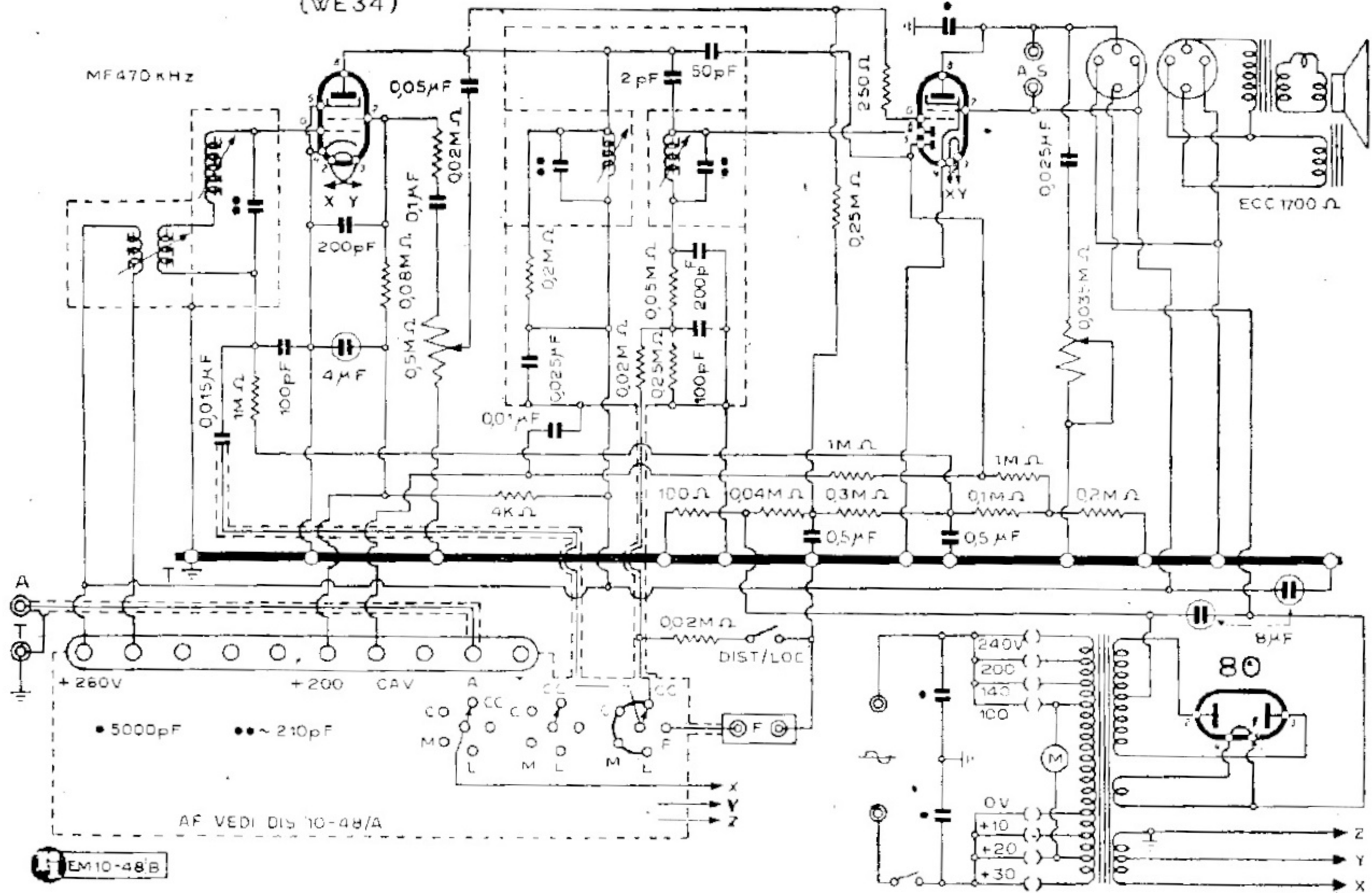
F.I.M.I. - MODD. PHONOLA « 505 » « 506 » - PARTE MF - RIV - BF - ALIM.
