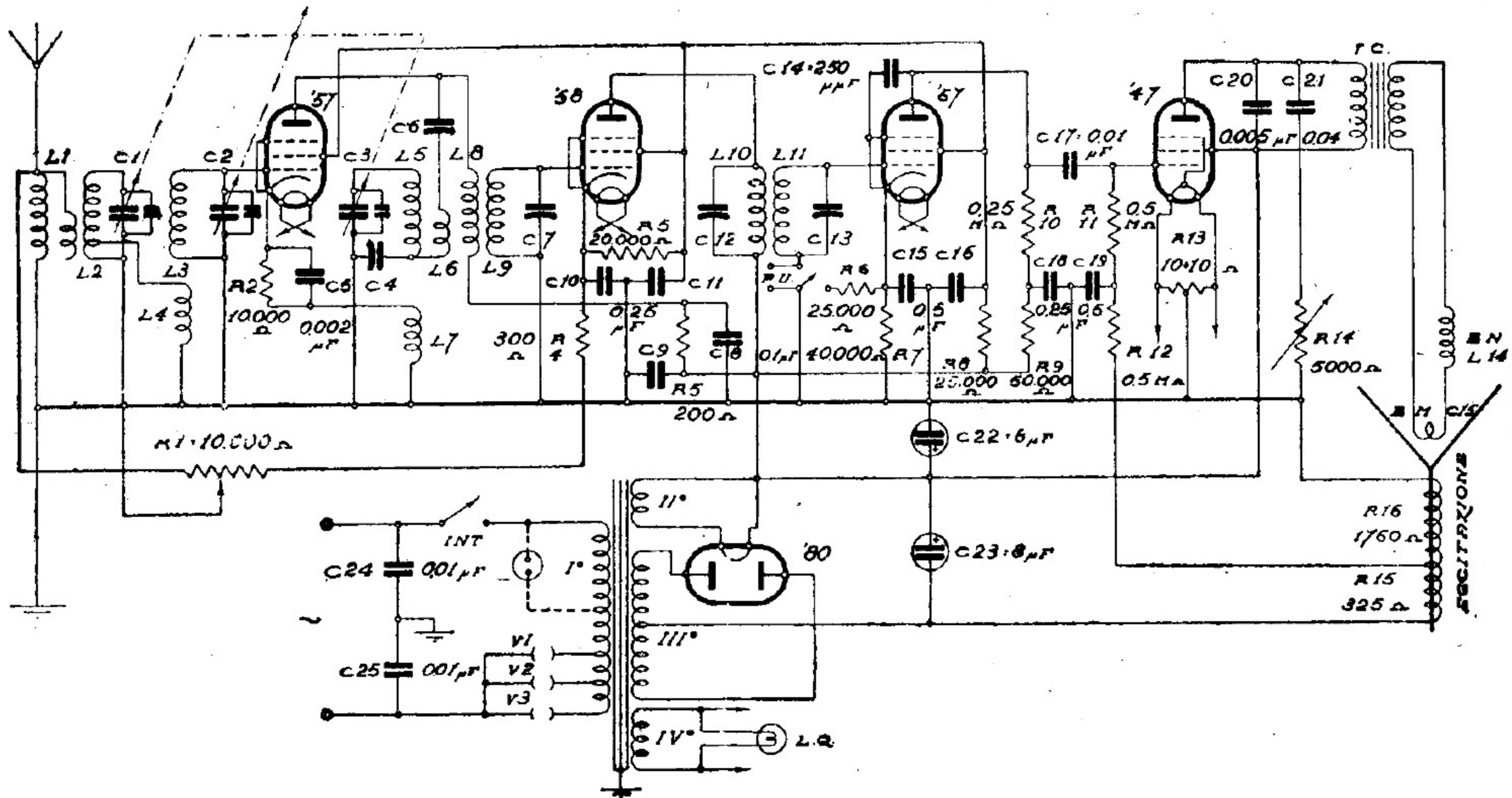
F.I.M.I. - MOD. PHONOLA « 581 » (ch. 560)
