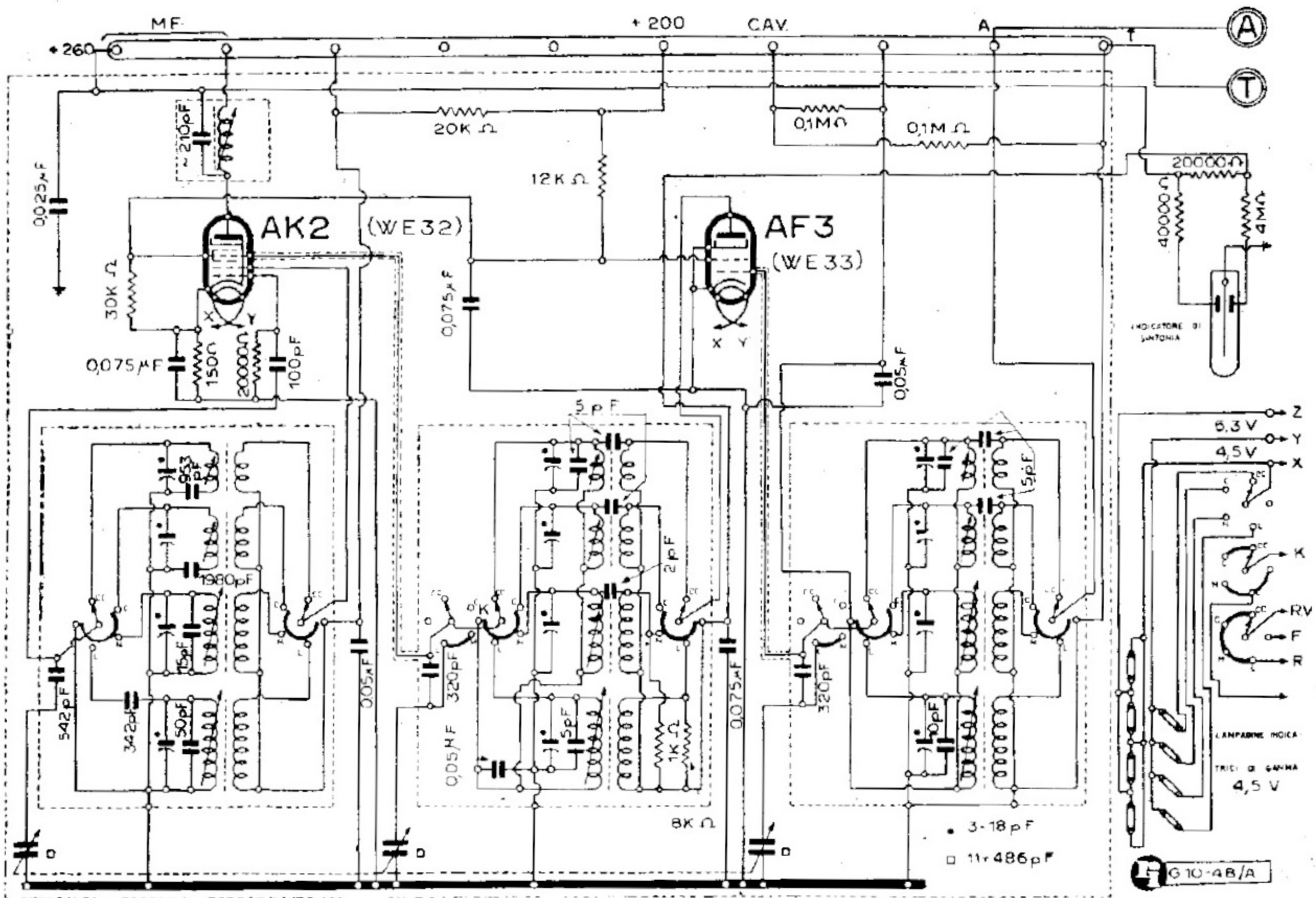
F.I.M.I. - MODD. PHONOLA « 605 » « 606 » - PARTE AF - CONV.
