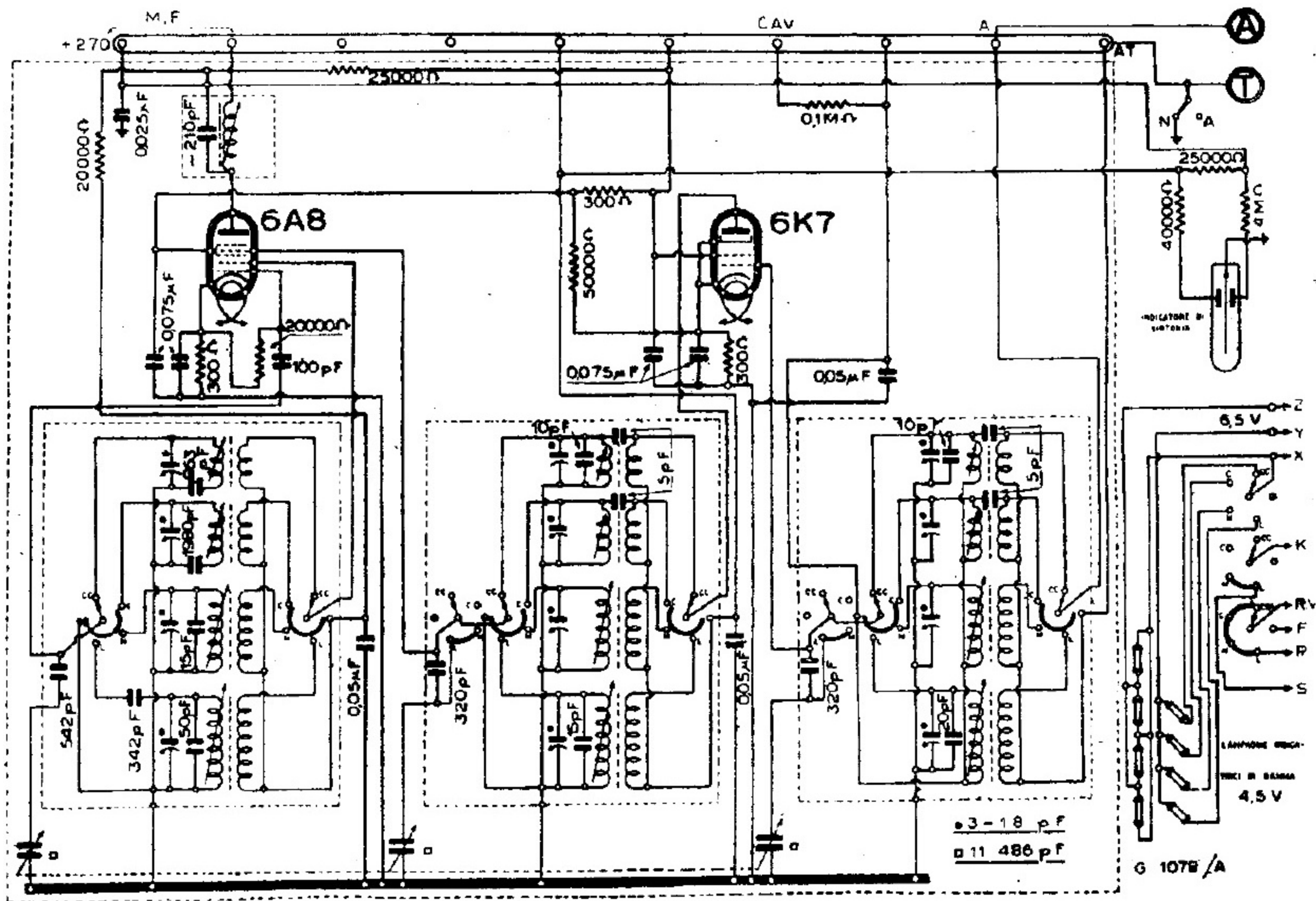
F.I.M.I. - MOD. PHONOLA « 880 » . PARTE AF
