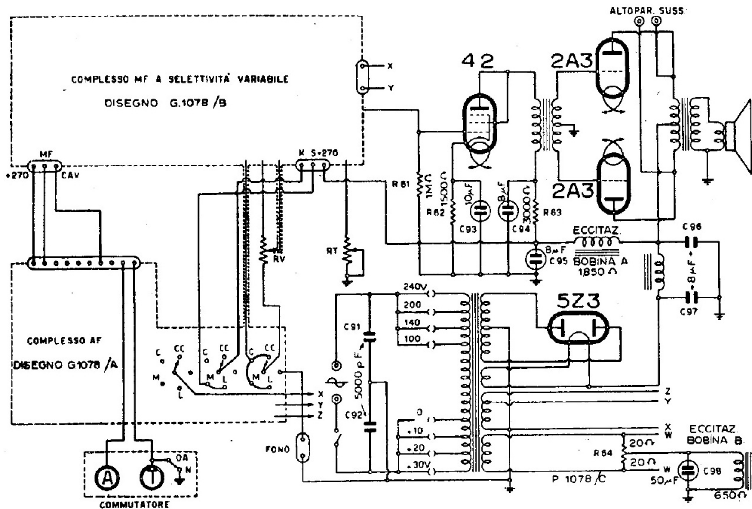
F.I.M.I. - MOD. PHONOLA « 880 » - PARTE BF
