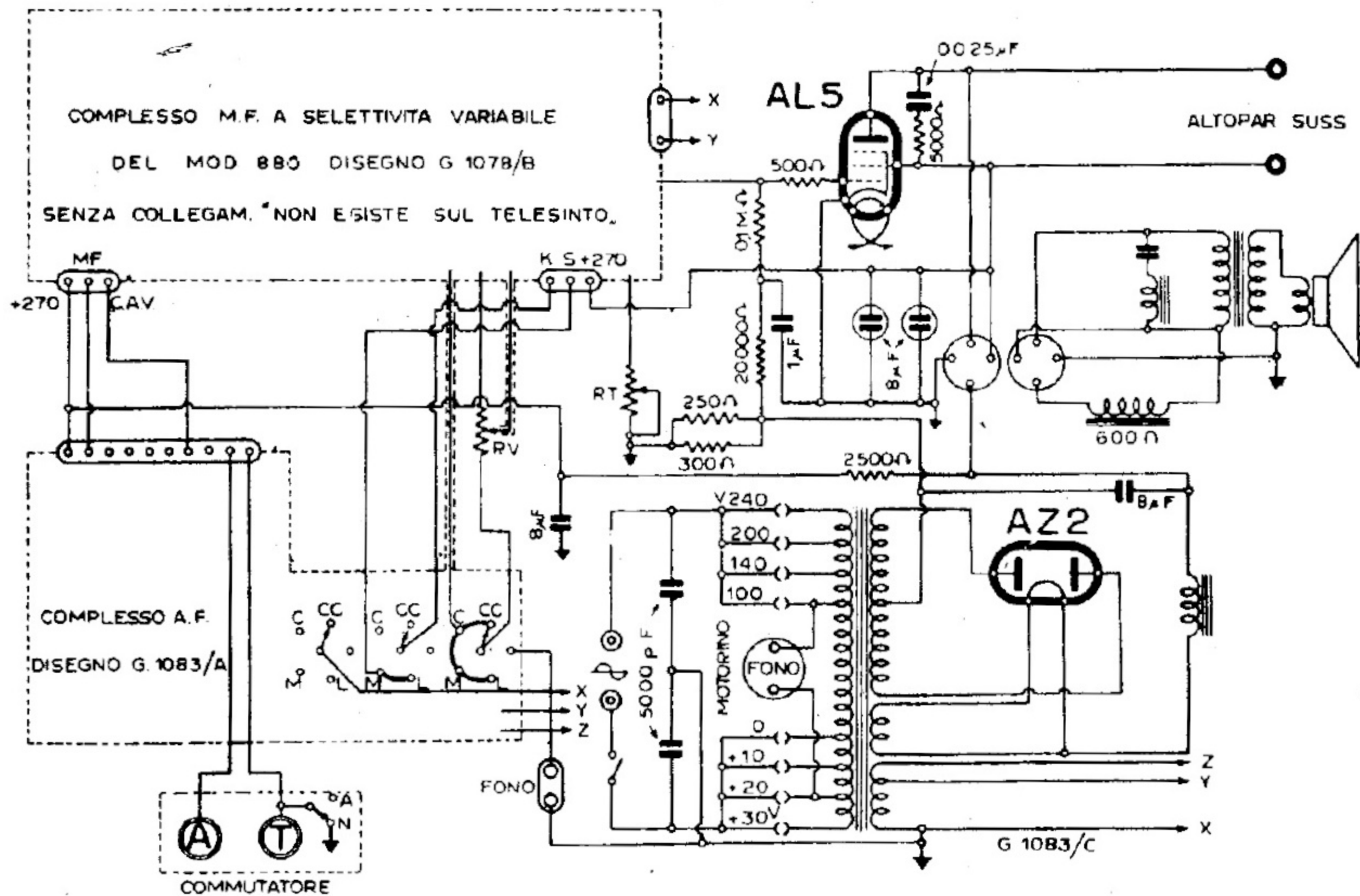
F.I.M.I. - MOD. PHONOLA « 960 » - PARTE BF
