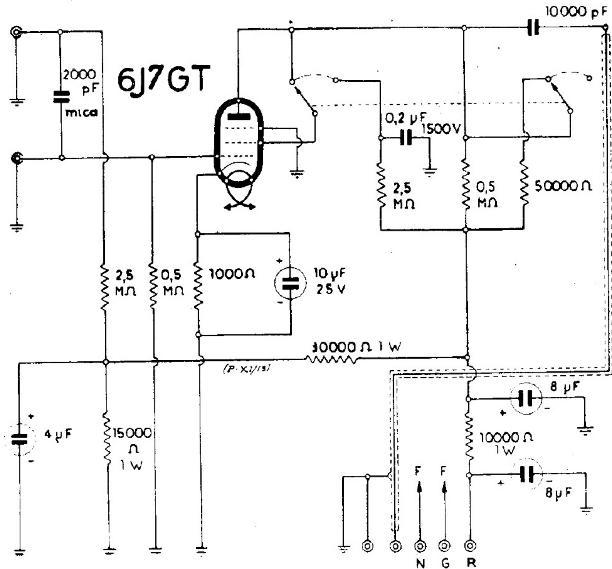
GALLO ING. G. - PREAMPLIFICATORE CONDOR - MOD. « PR1 »
