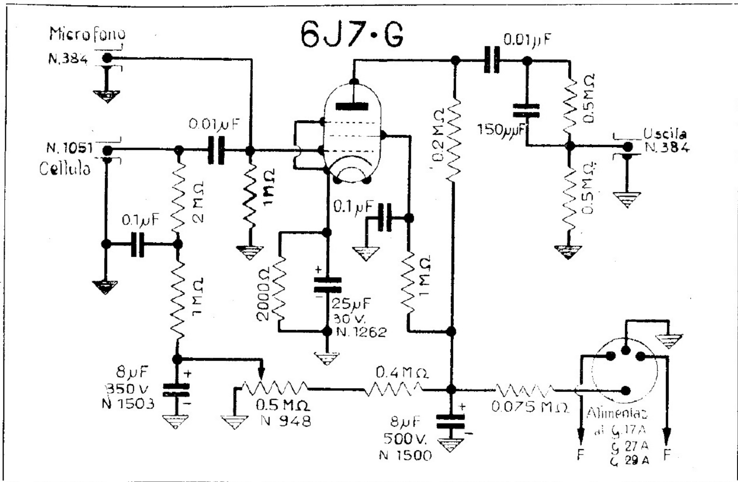
GELOSO (SOC.) - PREAMPLIFICATORE MOD. « G 1 »
