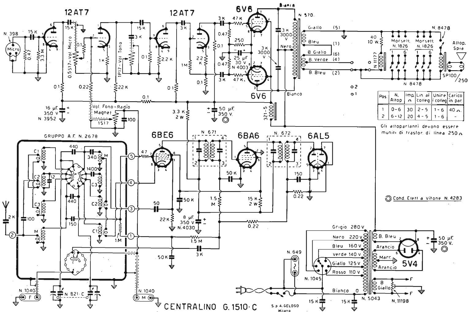
GELOSO - Mod. G. 1510-C - Ricevitore per dodici altoparlanti con potenza d'uscita complessiva di 15 watt. (Potenza di 12 W con 5 per cento di distorsione). Gamma onde medie e tre gamme onde corte. MF a 467 kc/s. Sensib. entr. microf.: 4 mV per piena potenza.
