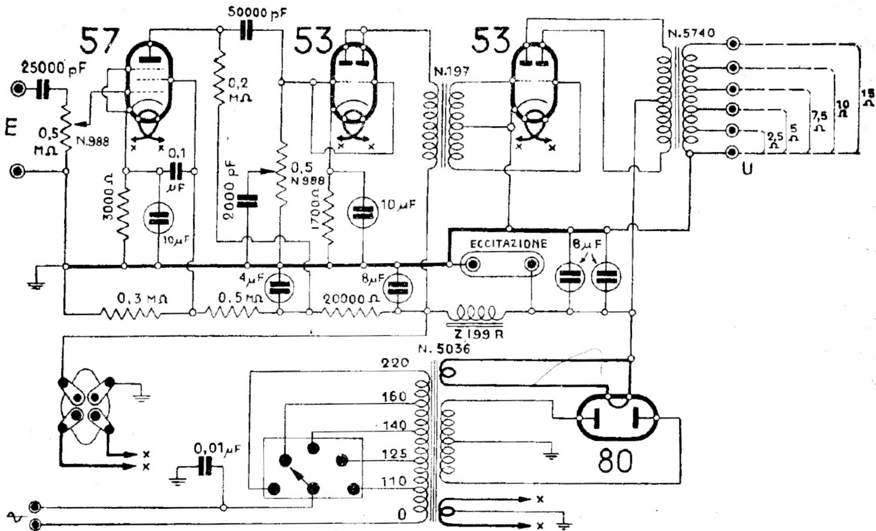
GELOSO (SOC.) - AMPLIFICATORE MOD. « G 17 A »
