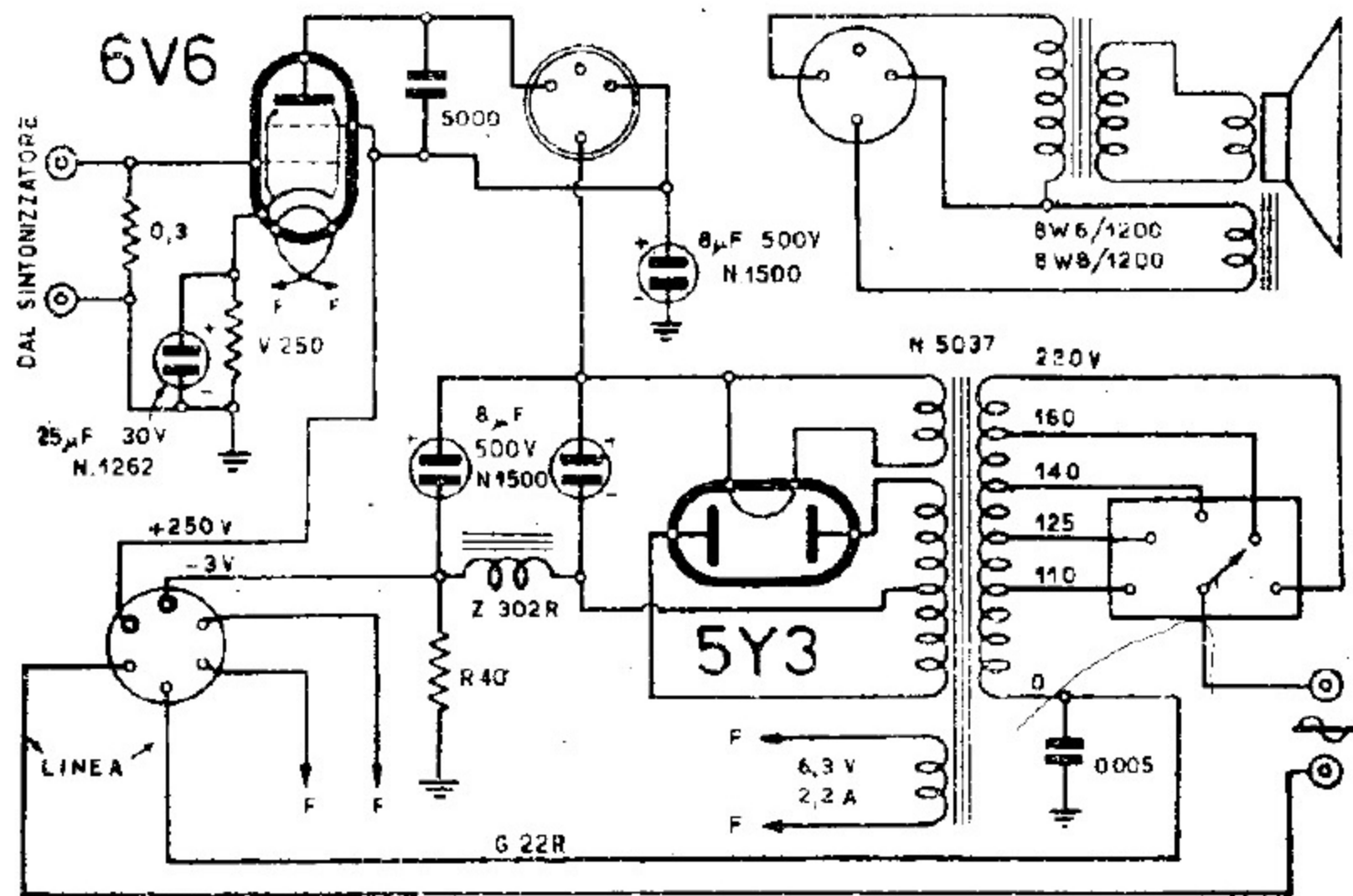
GELOSO (SOC.) - AMPLIFICATORE-ALIMENTATORE MOD. « G 22 R »
