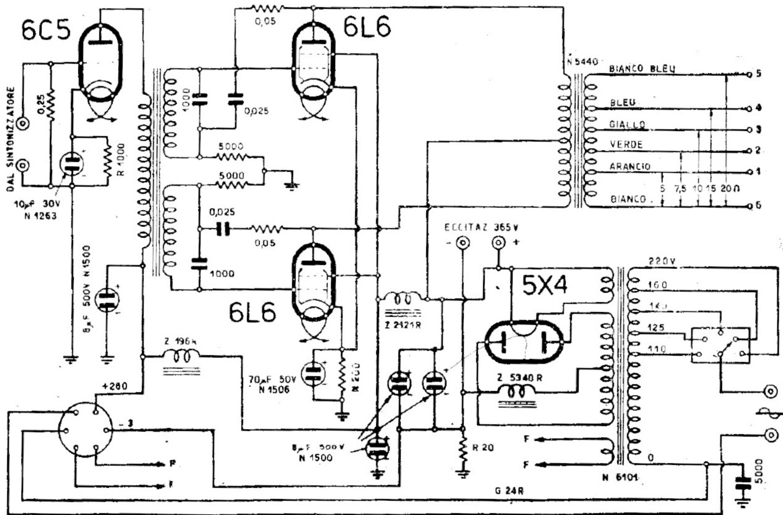
GELOSO (SOC.) - AMPLIFICATORE MOD. « G 24 R »
