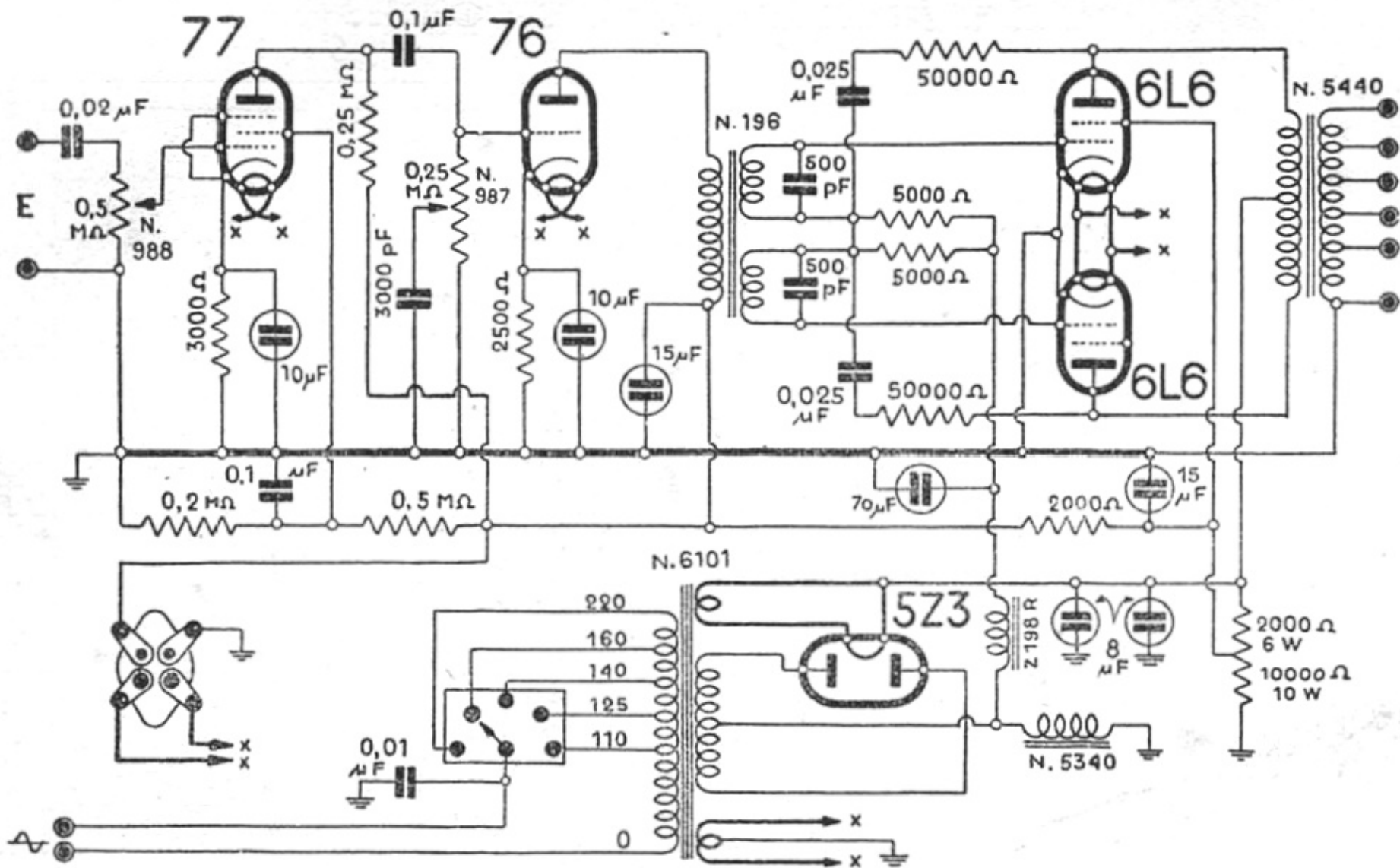
GELOSO J. S. A. - "AMPLIFICATORE G 27"
