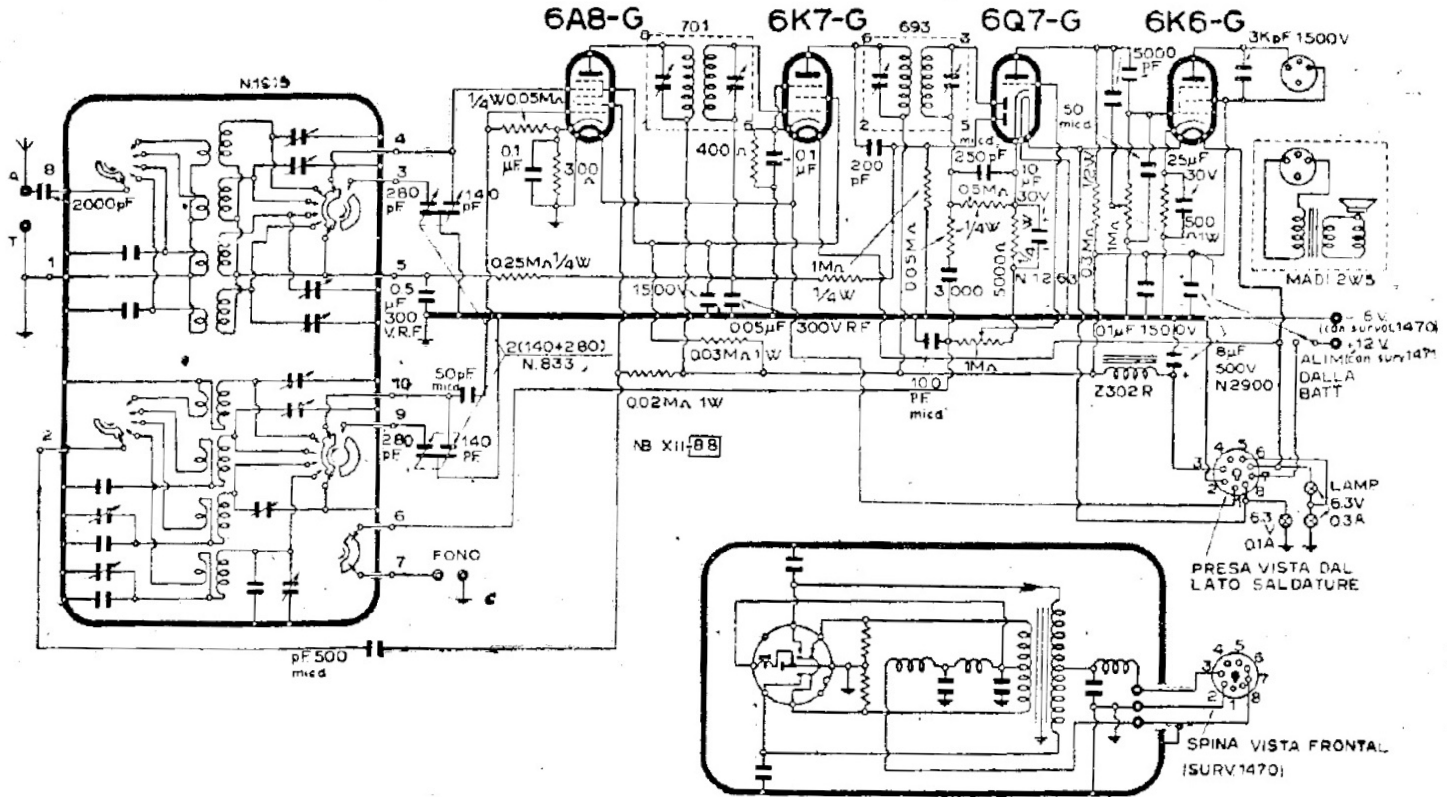
GELOSO (SOC.) - MOD. SUPER « G 49/A »
