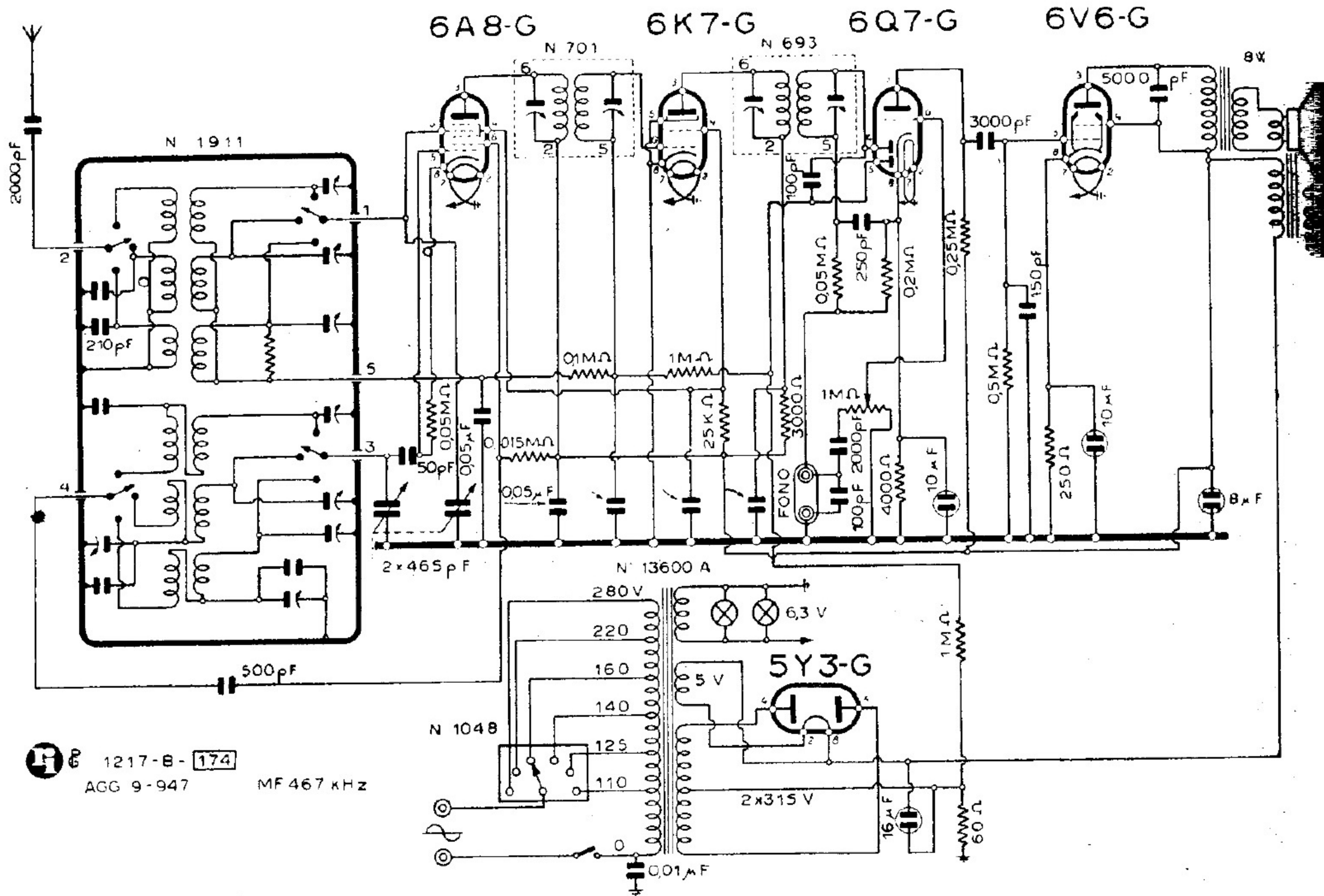
GELOSO (SOC.) - MOD. SUPER « G-51 » (Marzo 1945)
