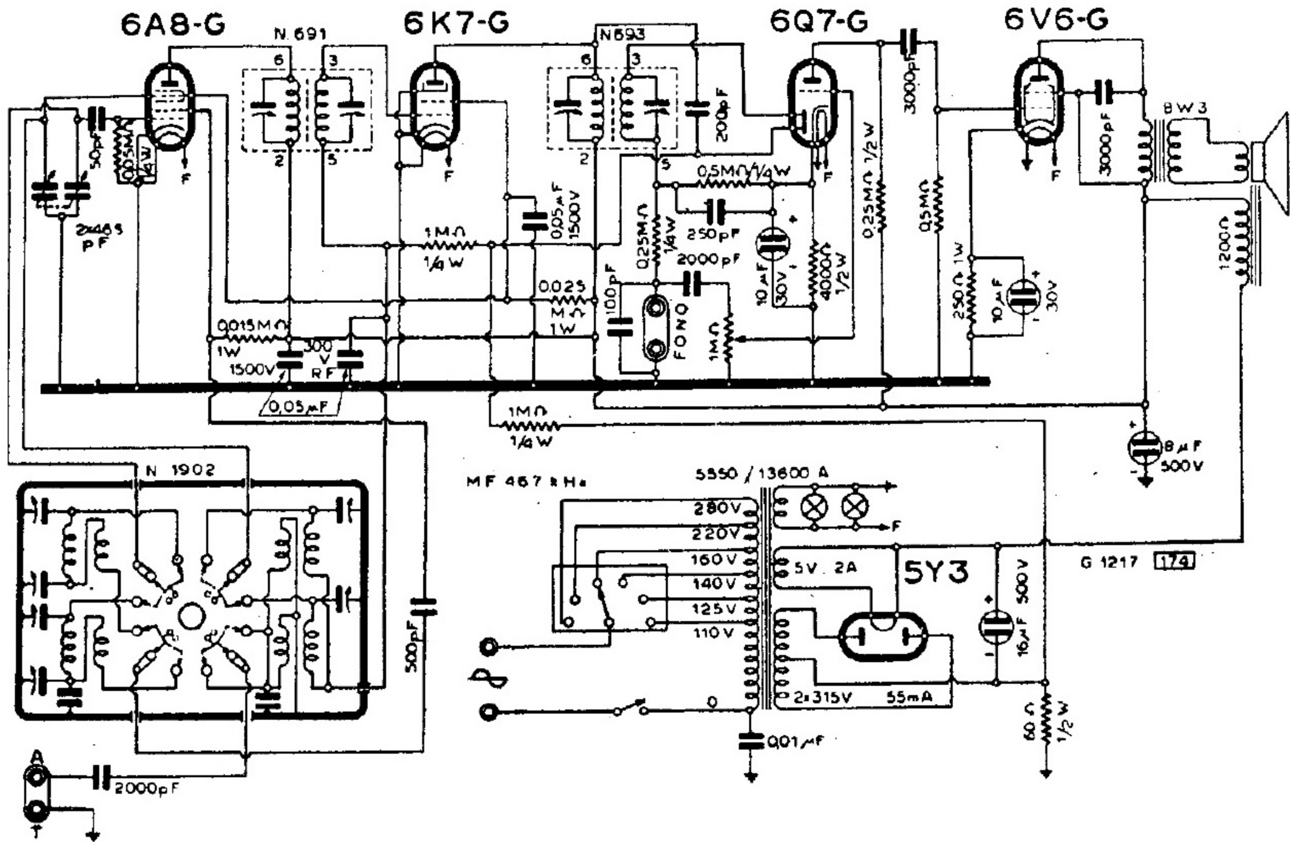
GELOSO (SOC.) - MOD. SUPER « G 51/44 »
