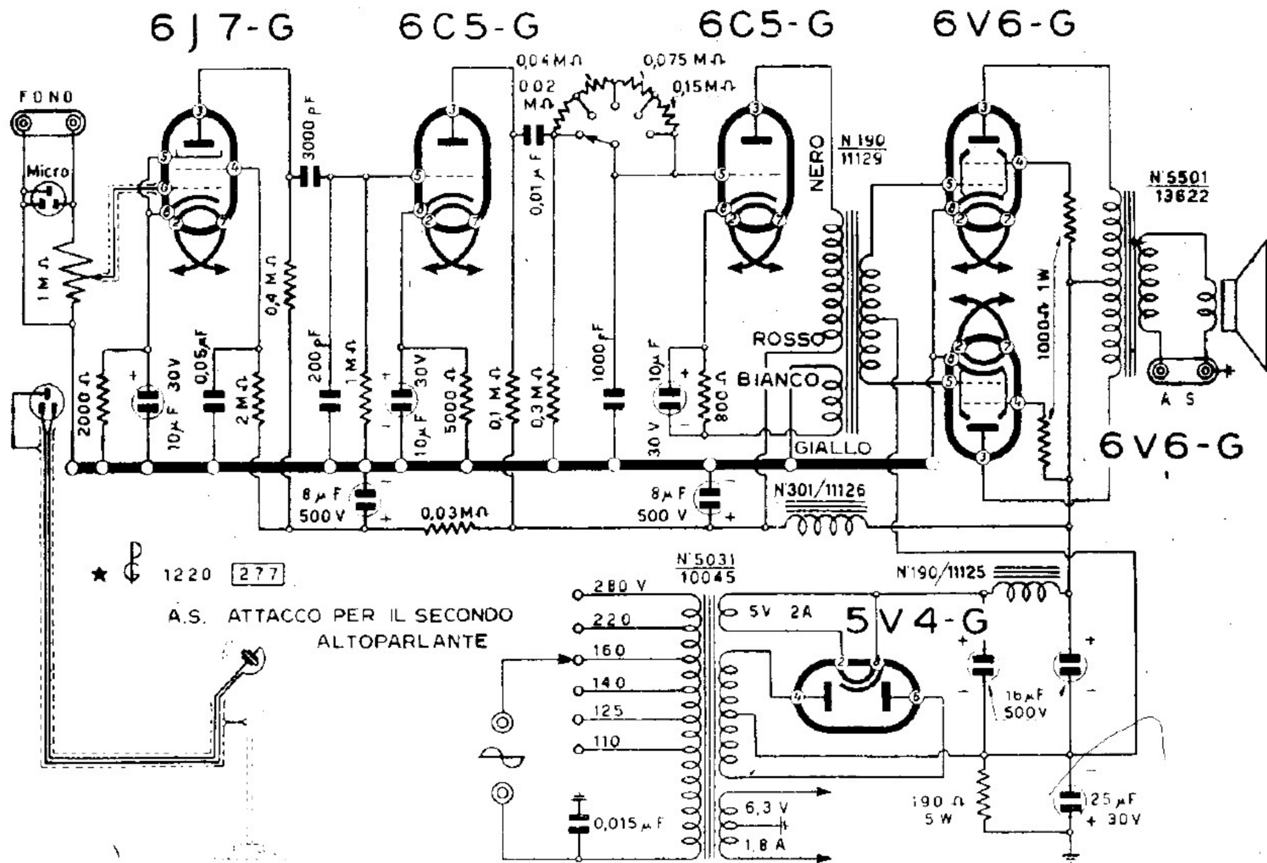
GELOSO (SOC.) - AMPLIFICATORE MOD. « G 5 V »
