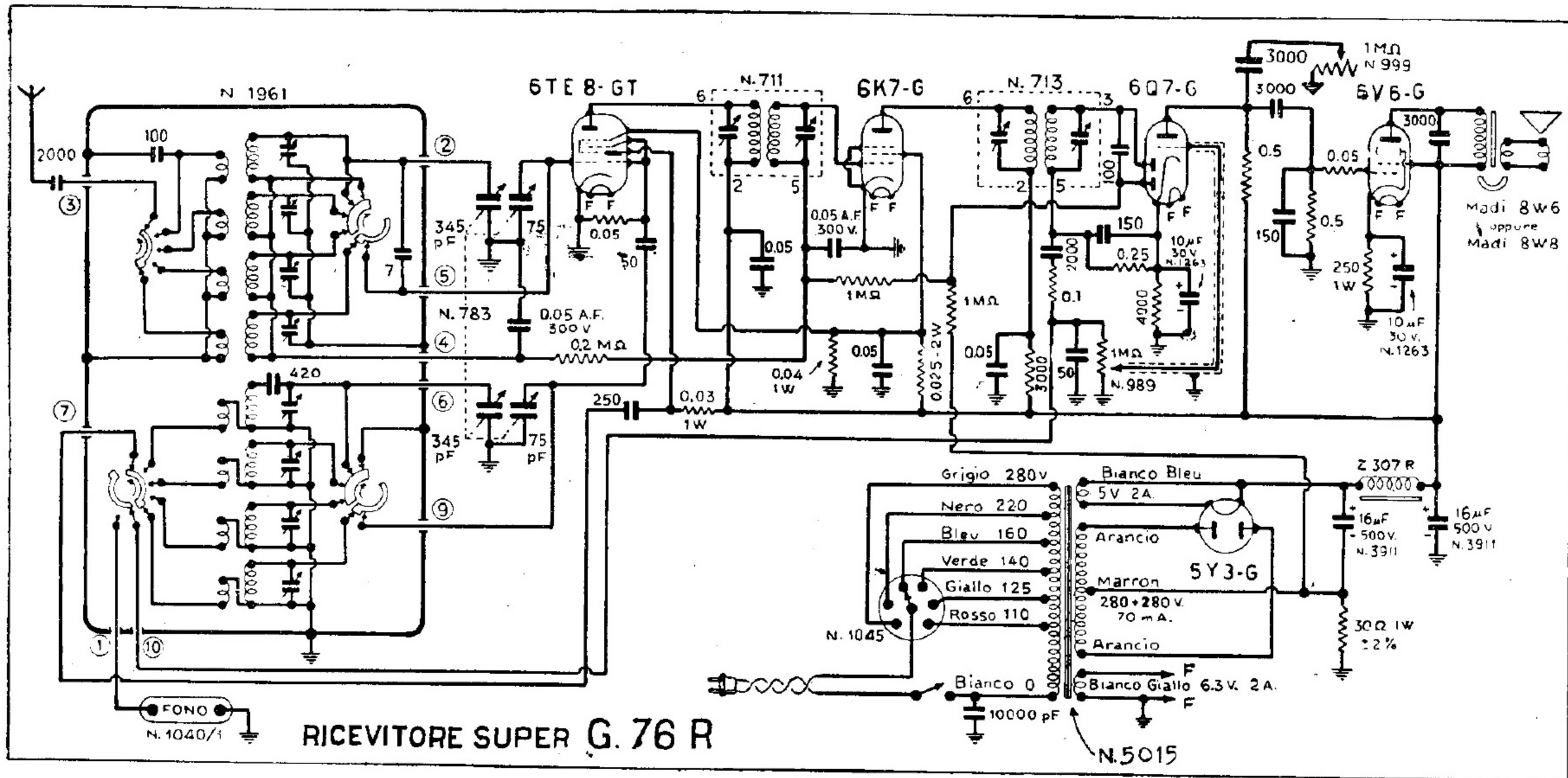
GELOSO (SOC.) - MOD. SUPER « G 76 R » (6TE8-GT)
