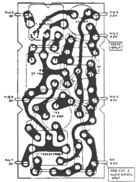
TOP VIEW IF MODULE (IM-5)
