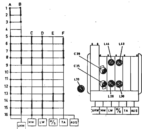
GRAETZ (Graetz Radio und Fernsehwerke, Altena) - Mod. Comedia 4R/216 - Apparecchio AM/FM a quattro gamme d'onda (lunghe, medie, corte) in AM e una banda in FM (onde ultracorte). Media frequenza AM a 472 ke/s, MF/FM a 10,7 Mc/s. Riproduzione, elettroacustica del tipo 3D, con un altoparlante magnetodinamico e due altoparlanti elettrostatici. Potenza d'uscita 4 watt indistorti. (Produzione 1956).
