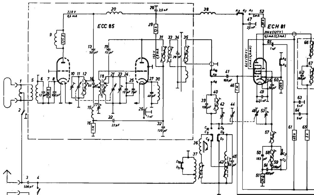
Musica 4R/217 GRAETZ KG. Altena
