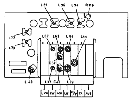
Chassis von unten gesehen
